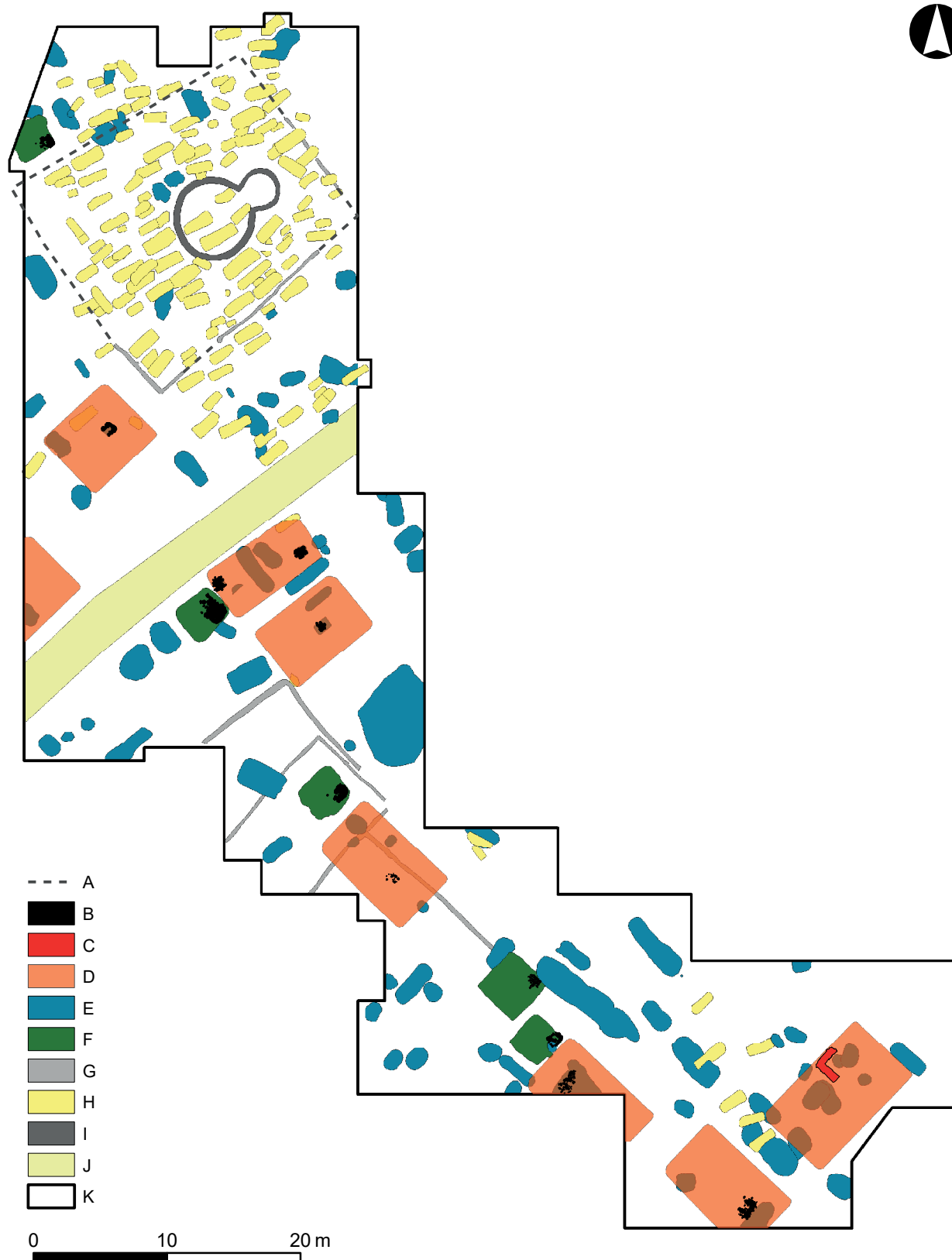
Obr. 142. Břeclav – Pohansko, Severovýchodní předhradí. Celkový plán funerální a sídlištní komponenty v okolí rotundy, výzkum 2008–2015. Legenda: A – rekonstrukce ohrazení, B – otopná zařízení, C – nároží zděné na maltu, D – předběžná rekonstrukce staveb založených na původním povrchu, E – ostatní zahloubené objekty, F – zemnice, G – žlábký ohrazení, H – ostatní hroby, I – základy kostela, J – předpokládaná komunikace, K – prozkoumaná plocha.
