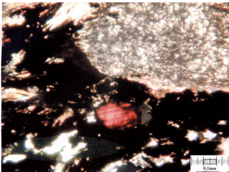
Obr. 7: Těšetice „Sutny“, surový grafit HD2, 1653 /0-20/, červenohnědý rutil v grafitové břidlici, XN, 10x.
