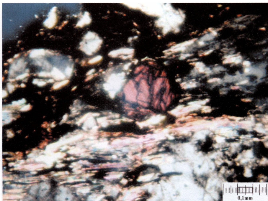
Obr. 4: Těšetice „Sutny“, grafitová keramika HD2, 1640B (60-80), červenohnědý rutil v grafitové břídlíci, XN, 10 \times .
