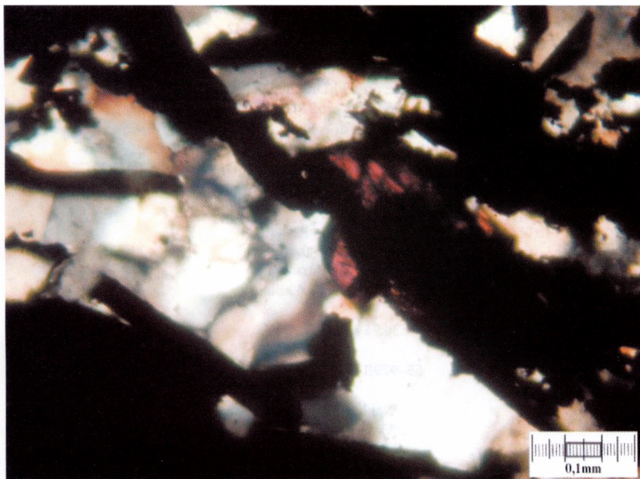
Obr. 8: Traisental, J II 72/266, surový grafit HD2 - 3, rutil v grafitové břidlici, XN, 10x.
