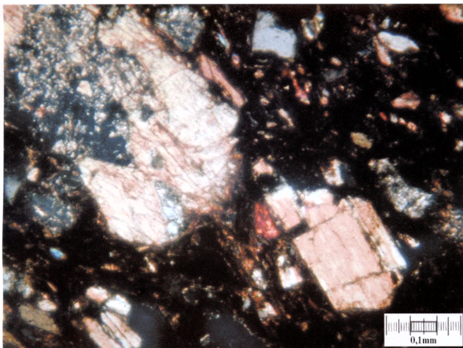
Obr. 3: Těšetice „Sutny“, grafitová keramika HD2, 1640A (100-130), zelené amfiboly a úlomky amfibolitových rul, XN, 10 \times .
