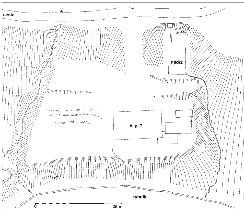
Obr. 2. Hradec, areál č. p. 7 – půdorysné zaměření. Stav v roce 2009. P. Kouřil, D. Prix.
