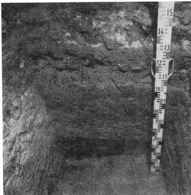
Obr. 3. Archeologická sonda v interiéri objektu Nálepka 16. V profile je v spodnej časti zreteľná základová rýha pre kamenný múr, zapustený 3 m do okolitého terénu. Horná valúnová dlažba pochádza zo 16.–17. storočia.
