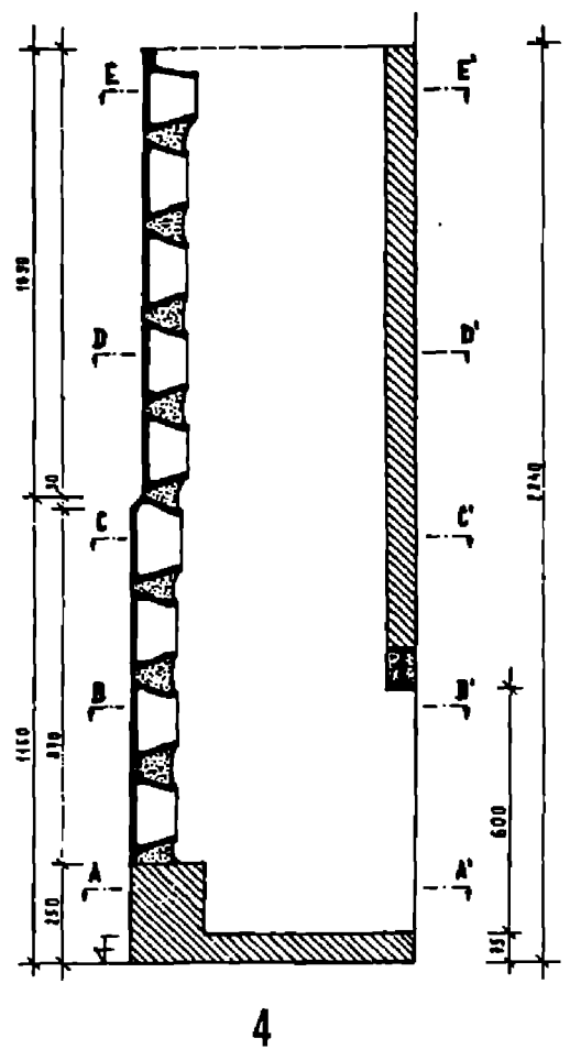
Obr. 6. Rekonstrukce pozdně gotických kamen z hradu Lichnice v MM Čáslav – stavební dokumentace. Nárys větší (1) a menší (2) boční stěny. Uvedená čísla kachlí odpovídají jejich obdobným číslům v textu. Svisté řezy stejných kamenných částí (3, 4). Kresba: M. Glosová.
