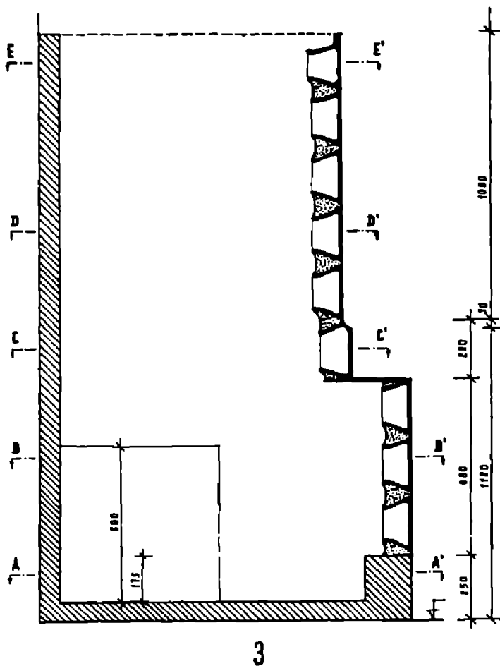
Obr. 6. Rekonstrukce pozdně gotických kamen z hradu Lichnice v MM Čáslav – stavební dokumentace. Nárys větší (1) a menší (2) boční stěny. Uvedená čísla kachlí odpovídají jejich obdobným číslům v textu. Svisté řezy stejných kamenných částí (3, 4). Kresba: M. Glosová.
