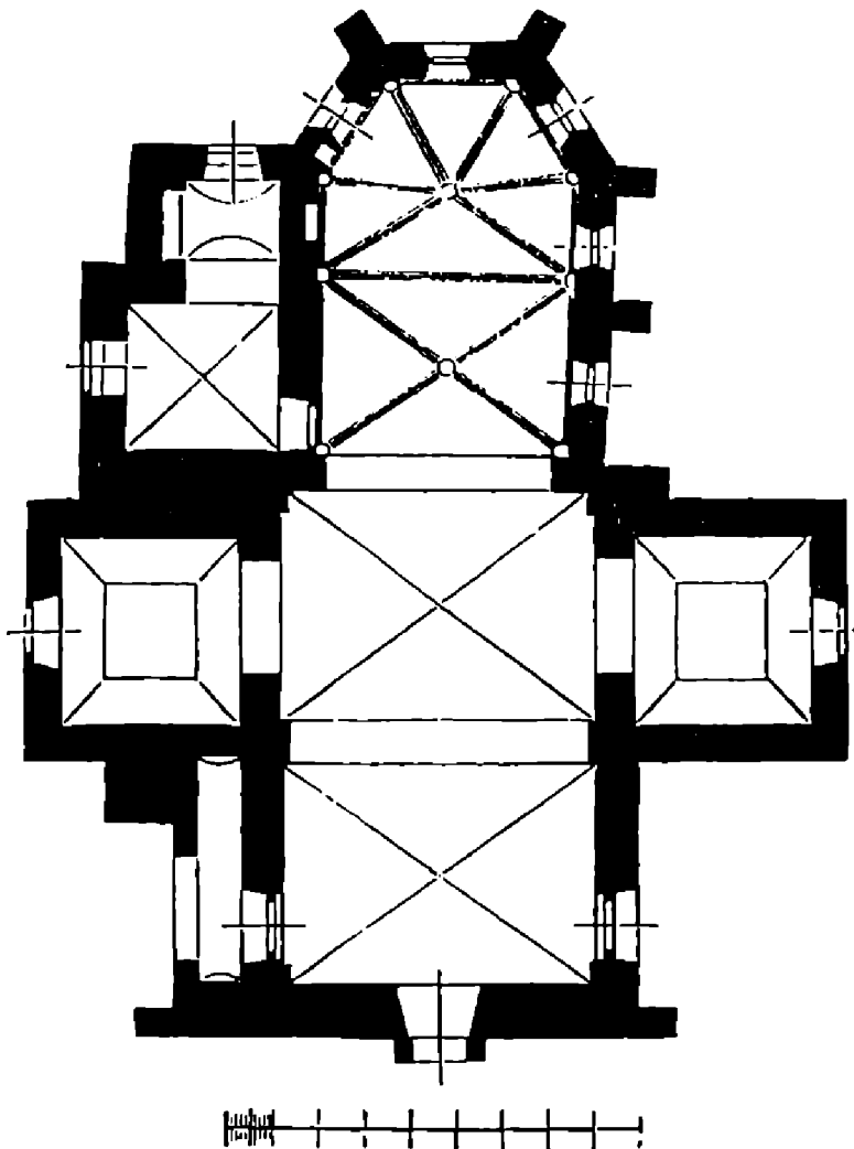
I. Trnava, špitálsky kostol sv. Heleny, pôdorys (podľa Henszlmanna).
