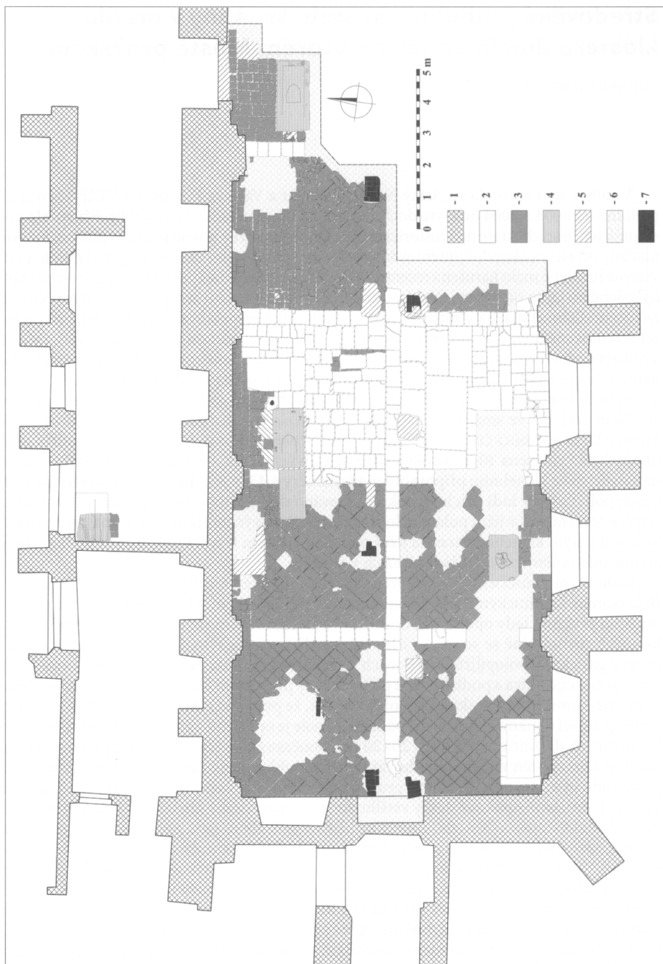
Obr. 1. Půdorys západní části kostela sv. Anny a jižního ramene ambitu se zaměřením středověké podlahy. 1 – zdivo kostela a klášterních budov, 2 – opuková dlažba, 3 – keramické dlaždice, 4 – kamenné náhrobní desky, 5 – maltová lože, 6 – zemina zásypů, 7 – novodobé cihly. Kresba J. Vachuda.
