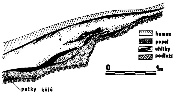
DETAIL STRATIGRAFIE FORTIFIKACE II
