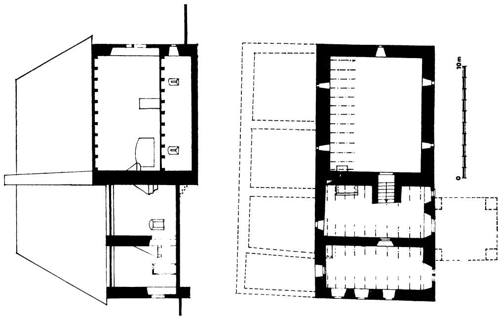
Obr. 4. Parížovce, kašiel. Grafická rekonštrukcia stavu kúrie po roku 1480. Kreslil M. Krizan.
