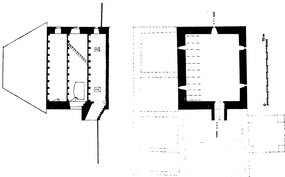
Obr. 3. Parižovce, kaštieľ. Grafická rekonštrukcia stavu kúrie z prvej polovice 14. storočia. Kreslil M. Krížan.
