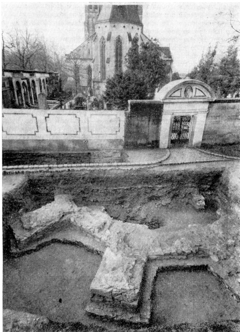
Obr. 2. Pohled od východu na objevené zdivo pětibokého gotického závěru s opěrnými pilíři a se soklovými díly svazkových hruškovitých přípor ze 14. století.
