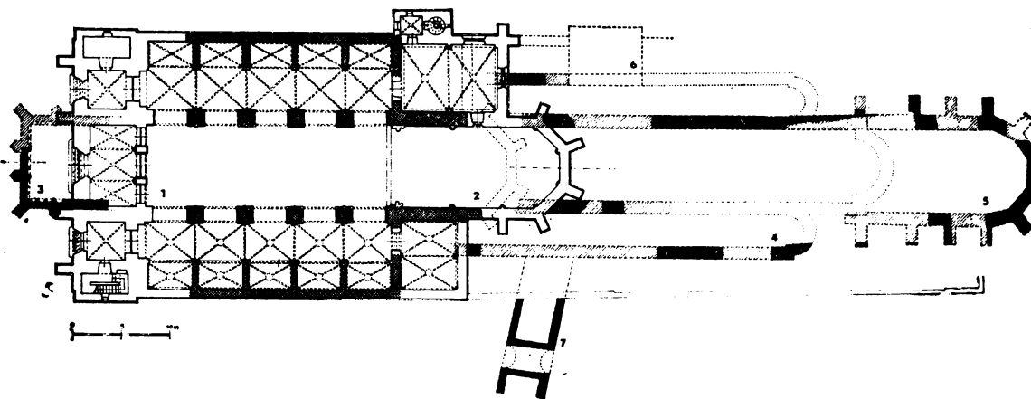
Obr. 1. Půdorys kostela sv. Petra a Pavla na Vyšehradě v rekonstrukci středověkého stavu na základě výsledků archeologického výzkumu: — řídké mřížky značí středověké zdivo nad terénem (včetně částí rekonstruovaných J. Mockerem) — husté mřížky — zaniklé středověké zdivo známé nebo zjištěné výkopem (včetně zdiva zjištěného v negativu), šikmá čára — dotvořený průběh zdiva mezi sondami. — 1 půdorys dnešního kostela, 2 — pozdně gotický případně renesanční kostelní závěr, zbořený při regotisaci, 3 — zaniklá gotická síň před západním průčelím kostela, 4 — nalezená apsida románské jižní lodi, 5 — závěr chrámu ze 14. století, 6 — situace bývalé zvonice.
