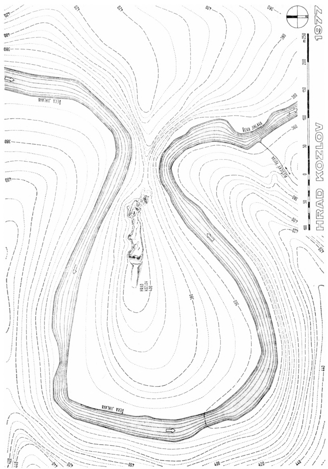
Obr. 1. Vrstečnicový plán okolí hradu.
