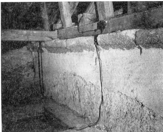
Obr. 3. Kostelec n/Vltavou (okr. Písek), kostel Narození P. Marie, podstřeší nad severní emporou. Pohled k východu podél horní části románské severní stěny lodi. Na koruně zdiva jsou díly tesané římsy, jejíž fabionový profil končil v místě, kde (na vzdálenějším konci stěny) přiléhá neomítané zdivo nad raně gotickým transeptem. Spodní část viditelného úseku románské stěny je rozrušena vybouráním arkády renesanční empory.
