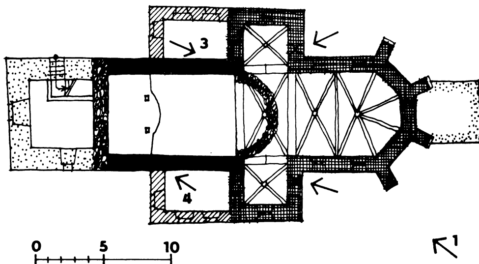
Obr. 2. Kostelec n/Vltavou (okr. Písek), kostel Narození P. Marie, schematický půdorys podle vyobrazení v Soupisě památek... (viz pozn. č. 1, str. 76) s analytickým vyznačením základních stavebních etap. Černě – dochované stěny románského kostela, kroužením doplněn předpokládaný průběh západního a východního ukončení. Křížkovane – raně gotický presbytář a příčná loď, šrafované – přístavba renesančních empor, tečkované – západní věž a východní sakristie. Šipky s čísly označují záběry snímků fotodokumentace, šipky bez čísel umístění druhotně zabudovaných románských oken.
