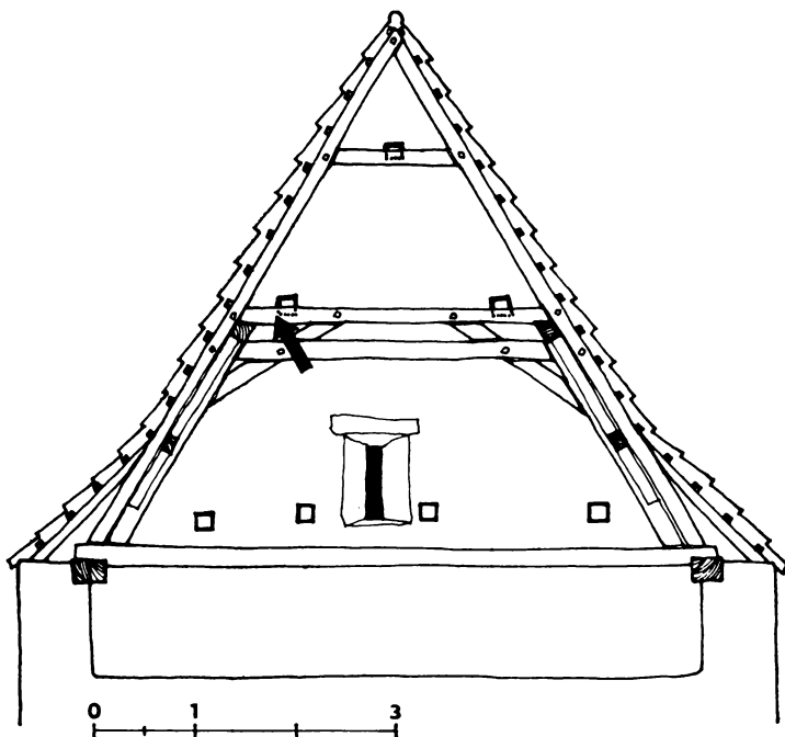
Obr. 2. Radošovice (okr. Strakonice), čp. 9. Pohled na vnitřní stranu západního štítu sýpky s vyznačením místa nálezu štěpů.
