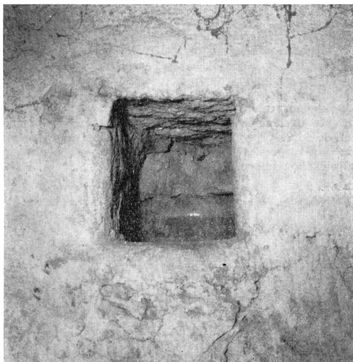
Obr. 8. Vochov (okr. Píseň-sever), žp. 10. Pohled do ústí skříže ve zdivu sýpky po vyjmutí uzavíracího kamene. V dolní části otvoru patrné hrdlo svísele zapuštěného, uvnitř hnědě glazovaného hrnce. (Foto a kresby J. Škabrada). Za upozornění na skříž děkujeme Vl. Svábkovi.
