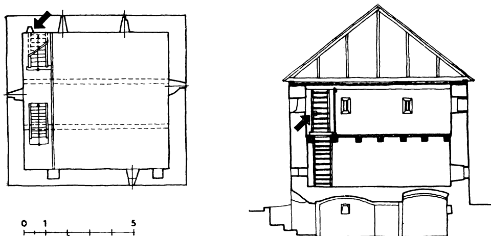
Obr. 5. Ostřetice (okr. Klatovy), čp. 14. Půdorys a řez sýpky s vyznačením umístění zazděné nádoby.
