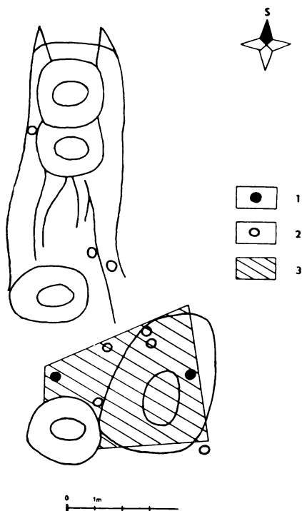
Obr. 3. ZSO Potálov, okres Tábor. Průzkum minohledáčkou Mi W 3 P. 1 – Předpokládaná místa nálezů kovů, 2 – anomálie, projevující se hlubším tónem, 3 – anomálie v ploše.
