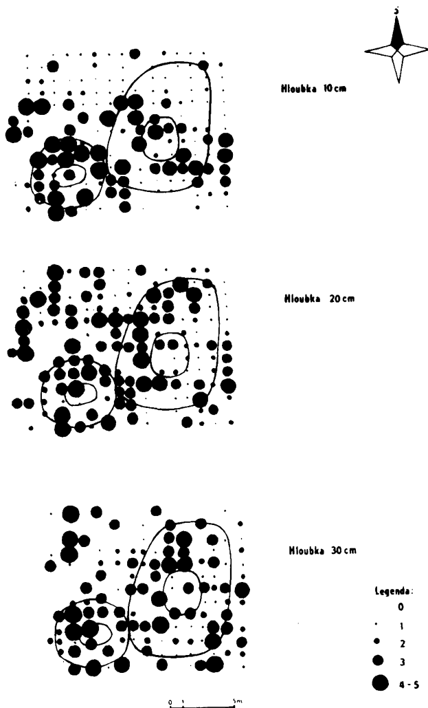
Obr. 4. ZSO Potálov, okres Tábor. Fosfátová analýza pomocí terenního testu v hloubkách 10–30 cm pod recentním povrchem. 0 — obsah 0,09 ‰–0,15 ‰ P_2O_5 , 1 — obsah nižší než 0,08 ‰ P_2O_5 , 2 — obsahy 0,16 ‰–0,4 ‰ P_2O_5 , 3 — obsahy 0,41 ‰–0,8 ‰ P_2O_5 , 4–5 obsahy vyšší než 0,8 ‰ P_2O_5 .
