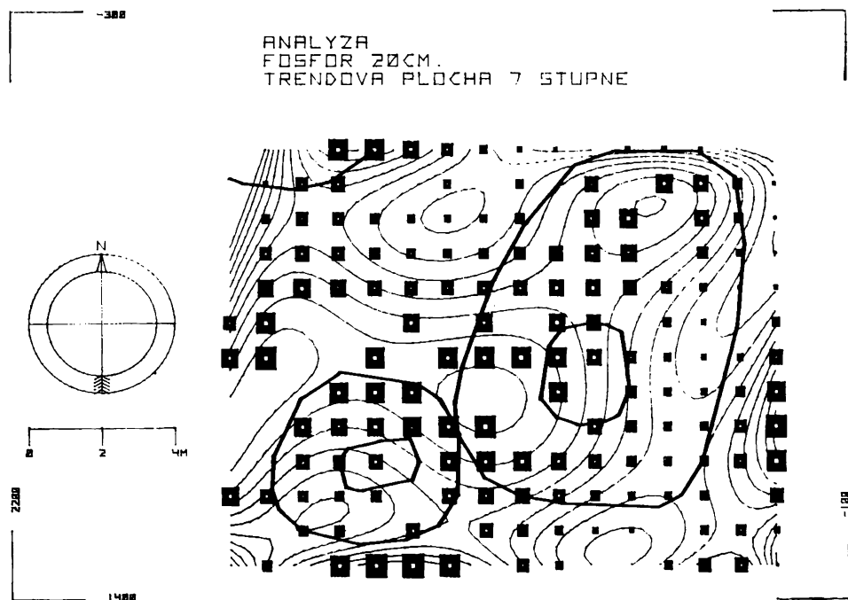
Obr. 8. ZSO Potůlův, okres Tábor. Trendová plocha 7. stupně proložená hodnotami obsahů P_2O_5 v hloubce 20 cm pod recentním povrchem.
