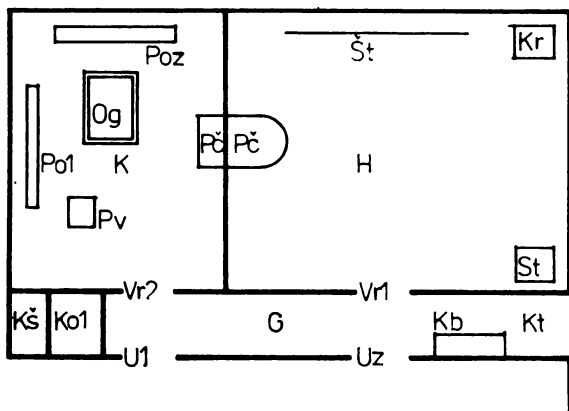
Obr. 7b. Vužjan, Chorvátsko. Hlavná obytná stavba rodiny Veliki Lucijanići: K – kuća, H – hiža, Vr1-2 – dvere, G – gánok, Ko1 – komorica, Kš – kurín, Kb – nádrž na pitnú vodu, U1,2 – vchody do gánku, Po1,2 – police, Pv – otvor do pivnice, Og – ohnisko, Pč – pec, Št – žrdka na sušenie odevu, Kr – krosná, St – stôl. V. Jurnić, 1960.
