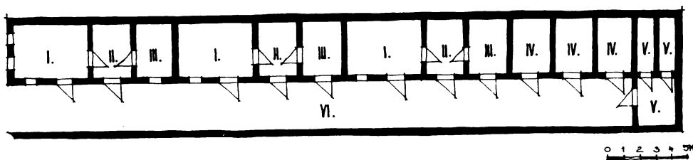
Obr. 13. Podkonice. Slovensko. Dlhý dom s tromi rezidenčnými jednotkami. I – izba, II – pitvor, III – komora, IV – mašťaľ, V – stodola, VI – dvor. A. Gregorčok Igovän, 1977.
