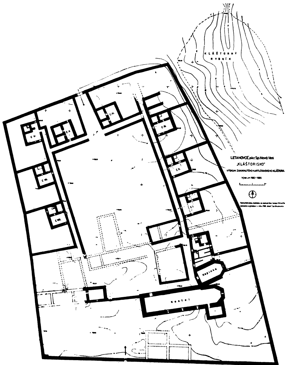
obr. 3. Predbežný pôdorys kartuziánskeho kláštora.
