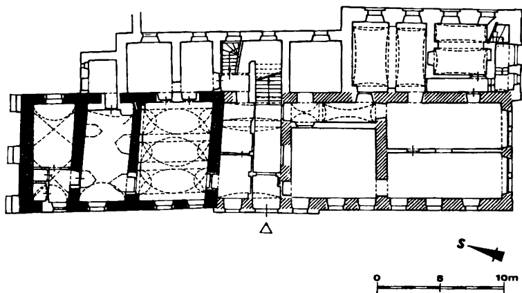
Obr. 19. Čkyně — půdorys přízemí dnešního zámku s dochovanými substrukcemi starší renesanční a barokní stavby.
