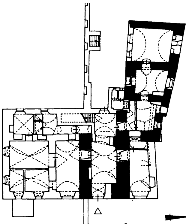
Obr. 8. Vlachovo Březí — půdorys přízemí dnešního zámku s dochovanými konstrukcemi středověkého hrádku.
