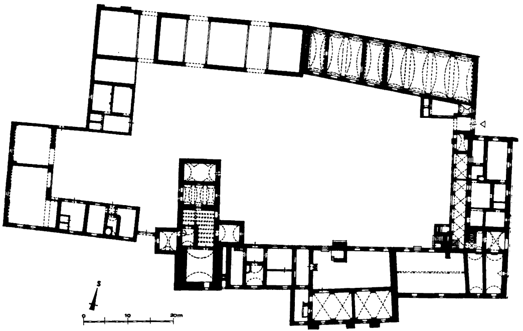
Obr. 20. Přečín — půdorys přízemí areálu zámku a dvorce na plánu z 2. pol. 19. století (doplňný o dochované klenby).
