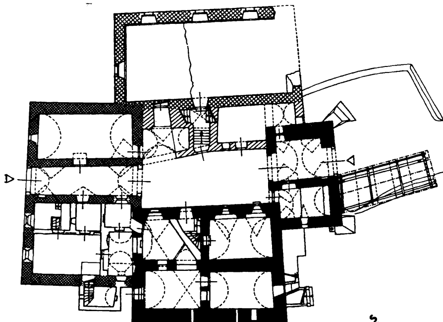
Obr. 13. Drslavice — půdorys přízemí bývalé tvrže.
