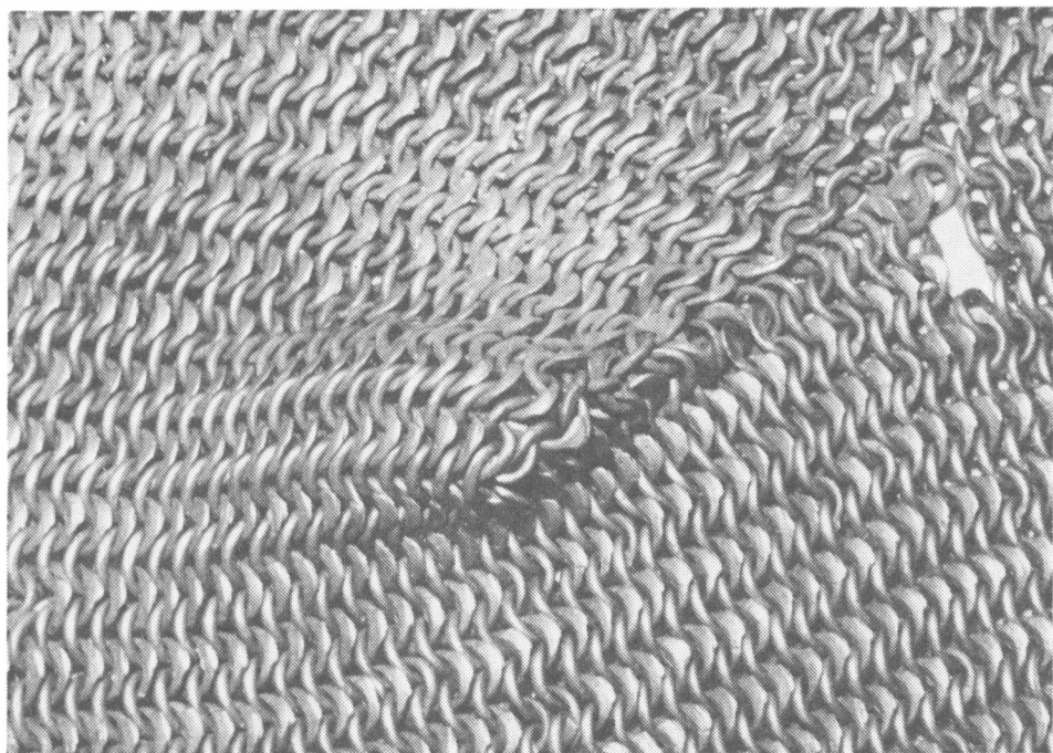
Obr. 3. Detail nejhustšího pletiva v oblasti brady (připojení roušky), pletivo typu „maglia ghiazzarina“.
