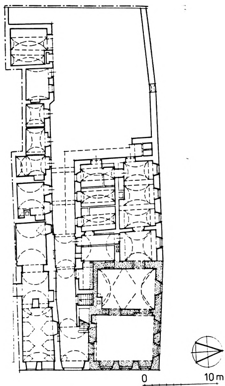
Obr. 7. Plzeň čp. 35, přízemí, tečkovaně označeno dvojičné jádro. — Kresby autor.
