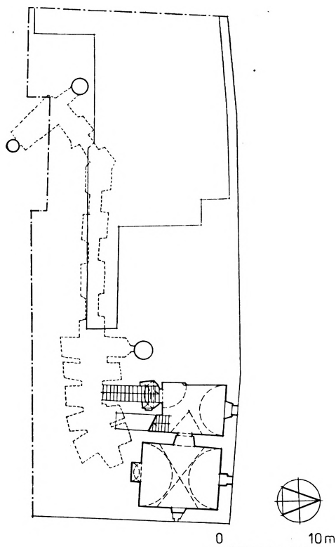
Obr. 6. Plzeň čp. 35, suterén, spodní sklepy čárkovaně.
