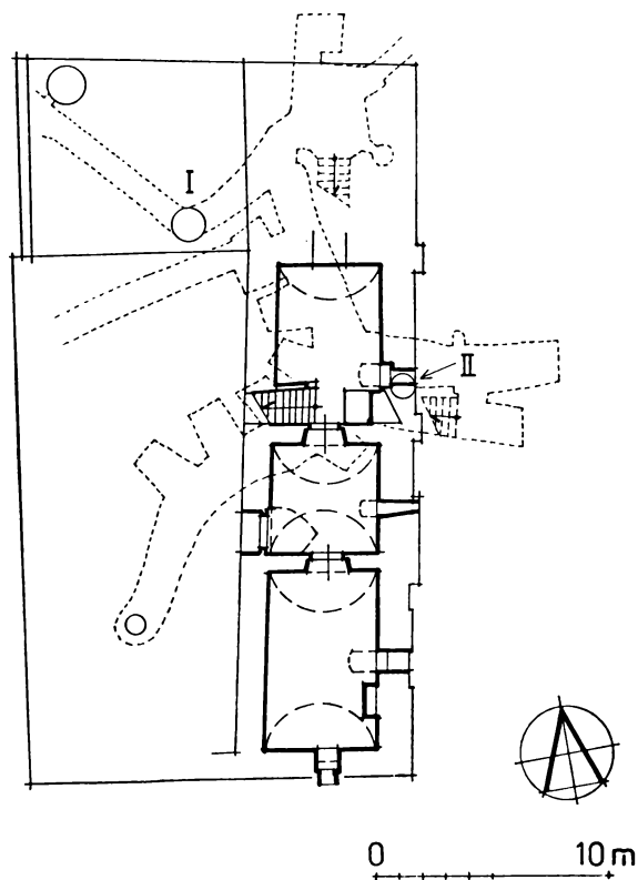
Obr. 2. Plzeň čp. 83, suterén, spodní sklepy čárkované.
