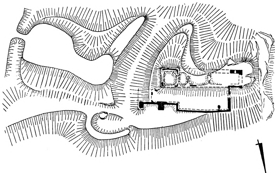
Obr. 12. Lapikus, terénní náčrt zříceniny.
