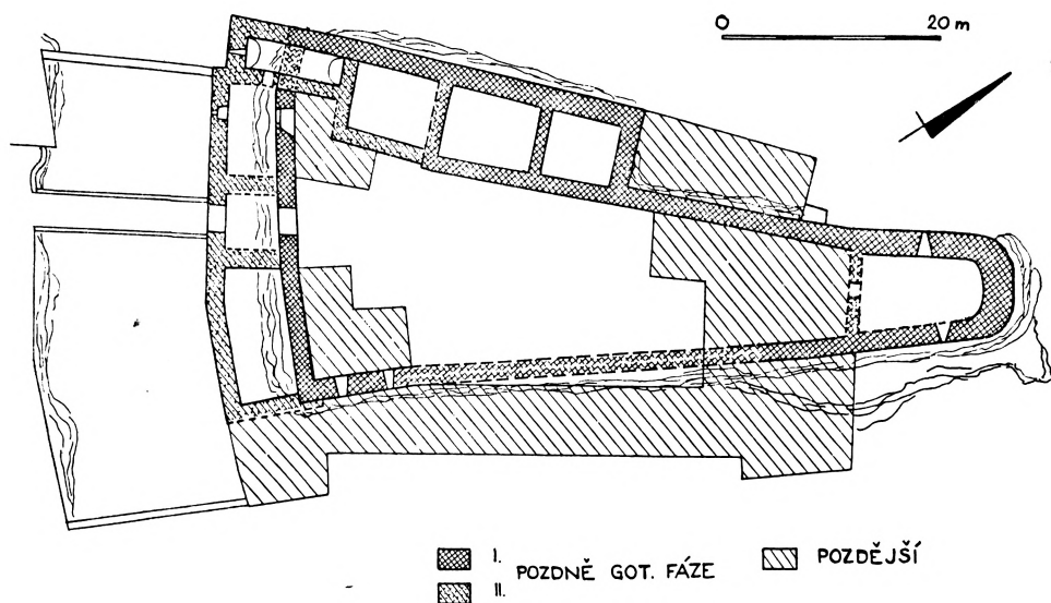
Obr. 14. Jevišovice-Starý zámek, pokus o vymezení nejstarší části zámku z pol. 15. stol. (křížkovně).
