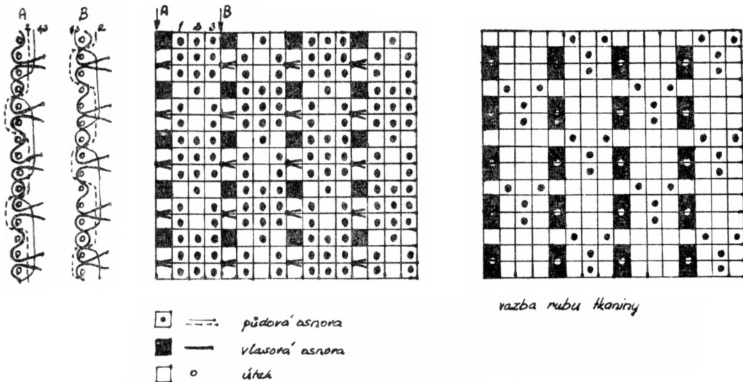
Obr. 2. Rozkres vazby sametu. Kresba A. Samohřívová.
