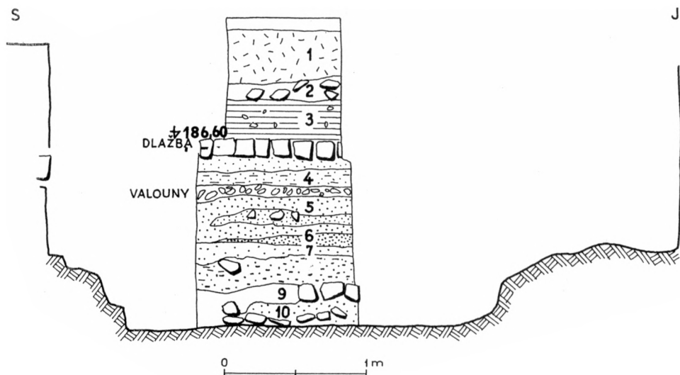
Obr. 8. Kostel sv. Šimona a Judy, sídlíštní objekt B/90 – řez S–J, pohled k východu: 1 – destrukce, 2 – opukové kameny, 3 – hlína s kameny a maltou, 4 – černý hlinitý písek, 5 – šedohnědá písčítá s uhlíky, 6 – šedohnědá písčítá, 7 – hnědý písek, 8 – hnědý písek s uhlíky a vápnem, 9 – hnědý písek s uhlíky, 10 – hnědý písek. Kresba: V. Huml.
