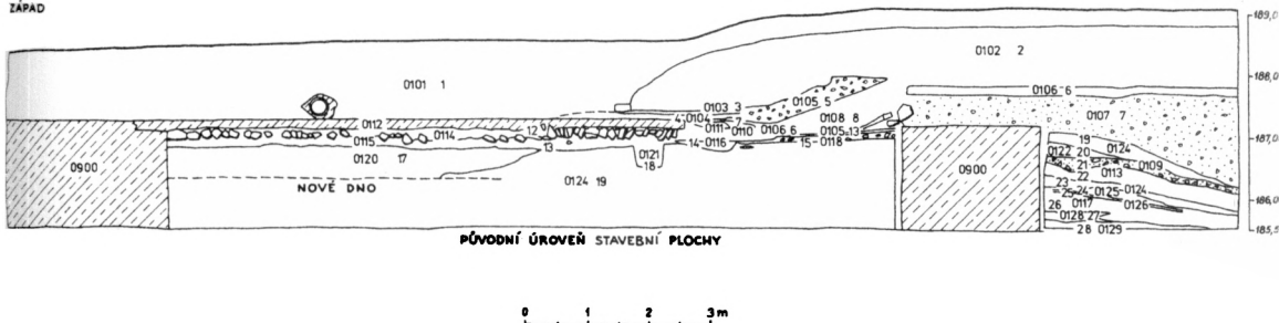
Obr. 6. Staveniště IHC (1992/93) – VZ směr, severní stěna: 1 – písčítá hlína, valouny, kameny, zl. cihel, 2 – hlinité závažky s velkými kameny, cihlami, 3 – tmavě šedá hlína, 4 – žlutý písek s valounky, 5 – drobné kaménky a štěrkůky, 6 – černá vrstva s uhlíky, 7 – hnědý písek, valounky, kaménky a zl. cihel, 8 – žlutý jíl, 9 – světle žlutý jíl, 10 – jilové písčítá, 11 – beton, 12 – velké kameny, 13 – tmavě šedá písčítá hlína, 14 – tmavě šedá hlinitá, 15 – štěrkůky, 16 – betonové základy university, 17 – hlinitý písek zl. cihel, kameny, 18 – tmavě šedá hlína, střeby oboustranně polévané, 19 – šedý popel, 20 – jemný zrnitý písek s kameny, 21 – prejzy, kameny a písek, 22 – šedý popel s uhlíky, 23 – šedohnědý popel, zbytky malty, 24 – šedý popel, 25 – tmavě šedá hlína s kaménky, 26 – šedý popel, zbytky malty, 27 – jíl s hnědým pískem se zbytky malty, 28 – tmavě šedý jíl s uhlíky. Kresba: V. Huml, M. Puk.
