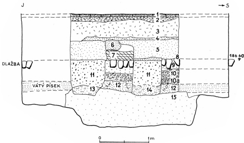
Obr. 9. Kostel sv. Šimona a Judy, profil S–J, západní strana: 1 – cihlové dlaždice, 2 – bílá vápnitá malta, 3 – stavební destrukce, 4 – šedý písek, 5 – šedohnědý jemný písek s částmi malty a vápnem, 6 – udusáný jemný zrnitý písek, 7 – šedohnědá hlína s kameny, 8 – opuková dlažba, 9 – světlý zrnitý písek, 10 – udusaná vrstva valounků prosypaných písekem světlehnědého odstínu, 11 – hnědý písčítý zásyp s drobnými kamenky, vápnítkými kusy a střepy keramiky, 12 – tmavě šedý písek s kusy kamenů, 13 – zásyp hrubou písčitohlinitý, odkryty 2 holenní kosti z kostry č. 12, 14 – šedý písčitohlinitý zásyp hrubou, 15 – hnědý písek s uhlíky, výplň obj. B/90. Kresba: V. Huml.
