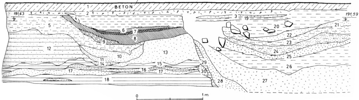
Obr. 2. Praha 1, Jilská ulice čp. 446/8. Řez terémem a pecí: 1 – beton, 2 – stavební suť, 3 – písek, 4 – jíl, 5 – hnědý hlinitý písek, 6 – okrová mazanice, 7 – tmavě šedý popel, 8 – kompaktní mazanice, 9 – červenohnědá rozdrobená mazanice, 10 – hnědožlutý mramorovaný písek, 11 – světle žlutý mramorovaný písek, 12 – světle béžový zrnitý písek s jílem, 13 – žlutý zrnitý písek, 14 – jíl s pískem, 15 – žlutý jíl, 16 – rezavý jíl s pískem, 17 – rezavý písek, 18 – žlutý mazlavý jíl, 19 – tmavě hnědá hlína, 20 – hnědá hlína s kameny, 21 – světle rezavý písek, 22 – světle šedý písek, 23 – světle šedohnědý písek, hlinitý, 24 – tmavě hnědá hlína s pískem, kameny a uhlíky, 25 – malta, zl. cihel, 26 – hnědá hlína s kameny, uhlíky, kusy malty a zlomky keramiky 16. stol., 27 – rozrušená malta, kusy cihel a kameny, 28 – světlá malta s kameny. Kresba: V. Huml.
