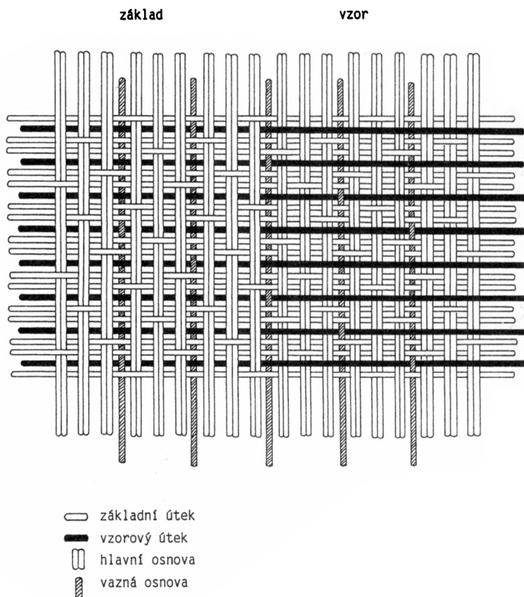
Obr. 3. Rozkres vazby tkaniny polštářku Matyáše z Arrasu. Kresba V. Otavská.
