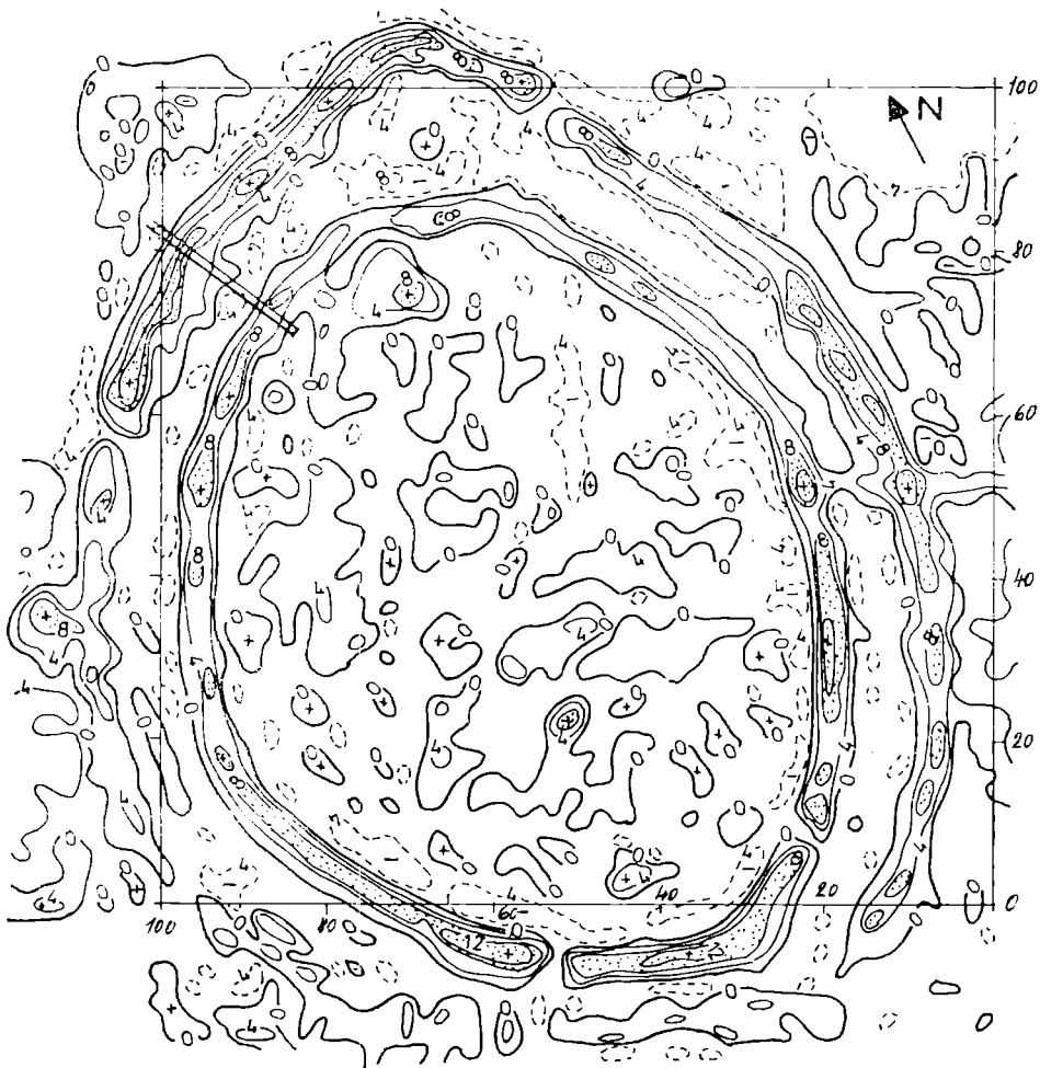
Fig. 1. Šumice, distr. of Znojmo. Map of \Delta T isoanomalies.
