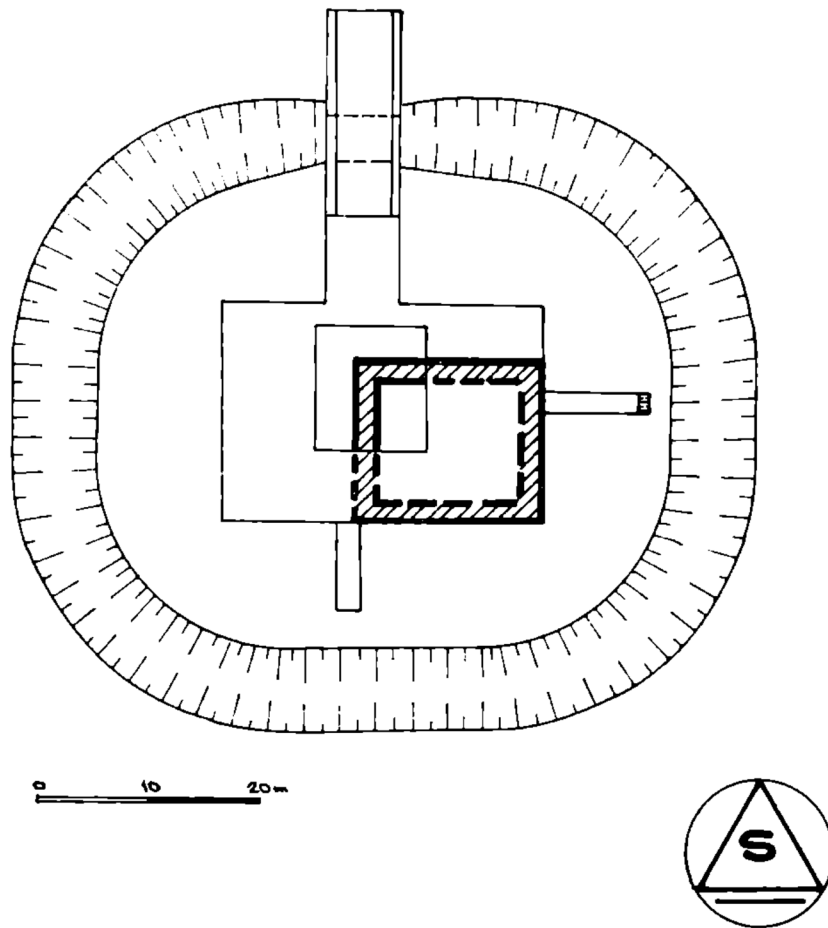
Obr. 1. Jeseník. Půdorys starší fáze tvrze.
