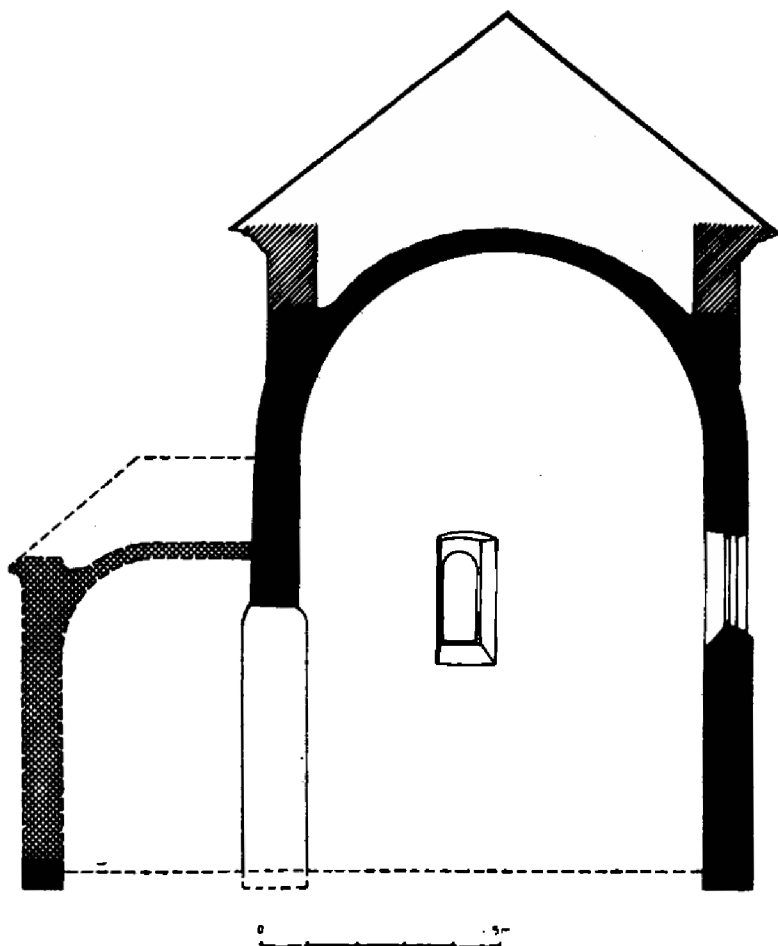
Obr. 3. Budeč, okr. Kladno, Ix stol. rotundou z 9./10. stol. doplněnou o objevenou východní apsidu (mřížka) a krov z 19. stol. (šikmá šrafa). Plná šrafa značí původní zachované zdivo
