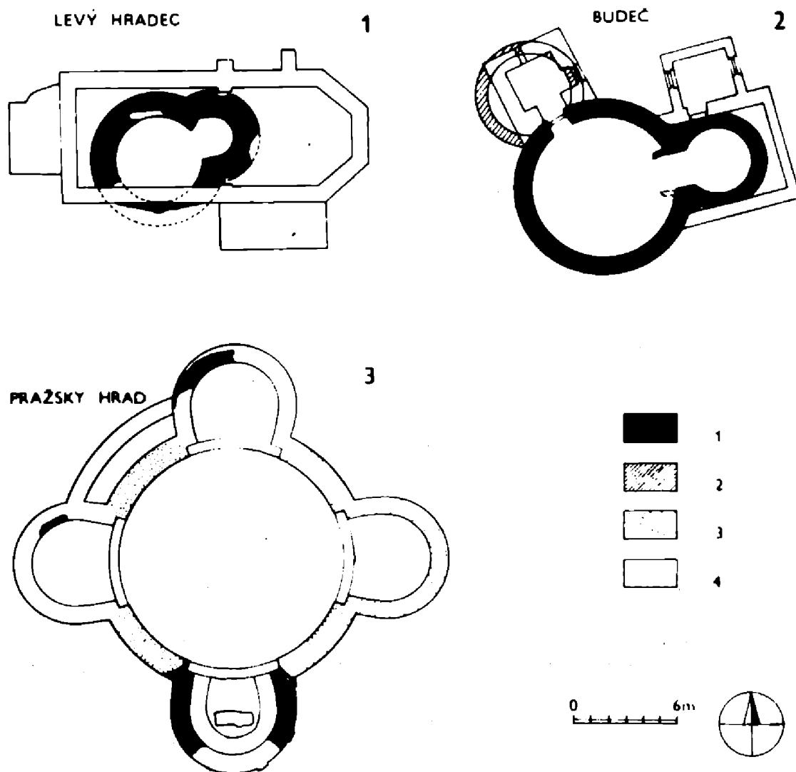
Obr. 4. Srovnání budečské rotundy (2) s Bořivojovou levohradeckou rotundou sv. Klimenta (9. stol.) a svatováclavskou centrálou na Pražském hradě (10. stol.). Šrafy – 1: zachované původní zdivo, 2: přistavěná hrobní kaple u budečské rotundy z 11. stol., 3: rekonstrukce svatováclavské centrály v půdorysu, o jejímž tvaru není pochyb, 4: pozdější stavební úpravy srovnávaných kostelů v gotice (1): v románské době, v baroku, (2): v partích, na něž není shodný názor odborníků (3).
