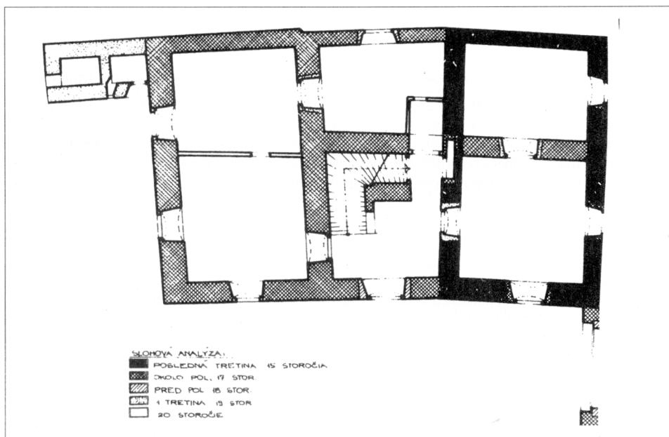
Obr. 11. Spišská Kapitula, pôdorys kanonického domu č. 5 s gotickým jadrom.
