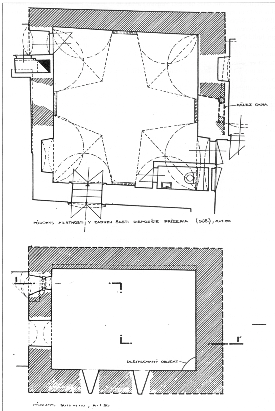
Obr. 2. Levoča, námestie č. 25, nálež jednopriestorového domu, suterén a prízemie.
