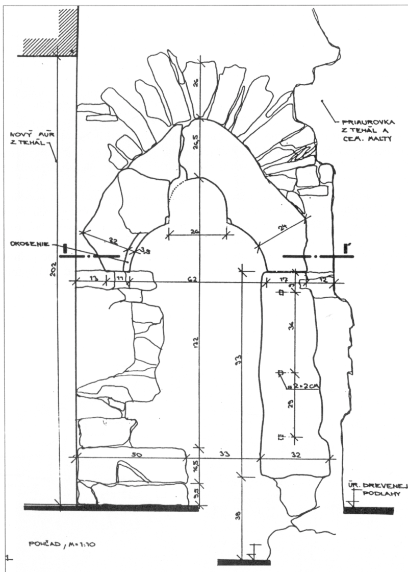
Obr. 3. Levoča, námestie č. 25, nálež okna s mníškou.
