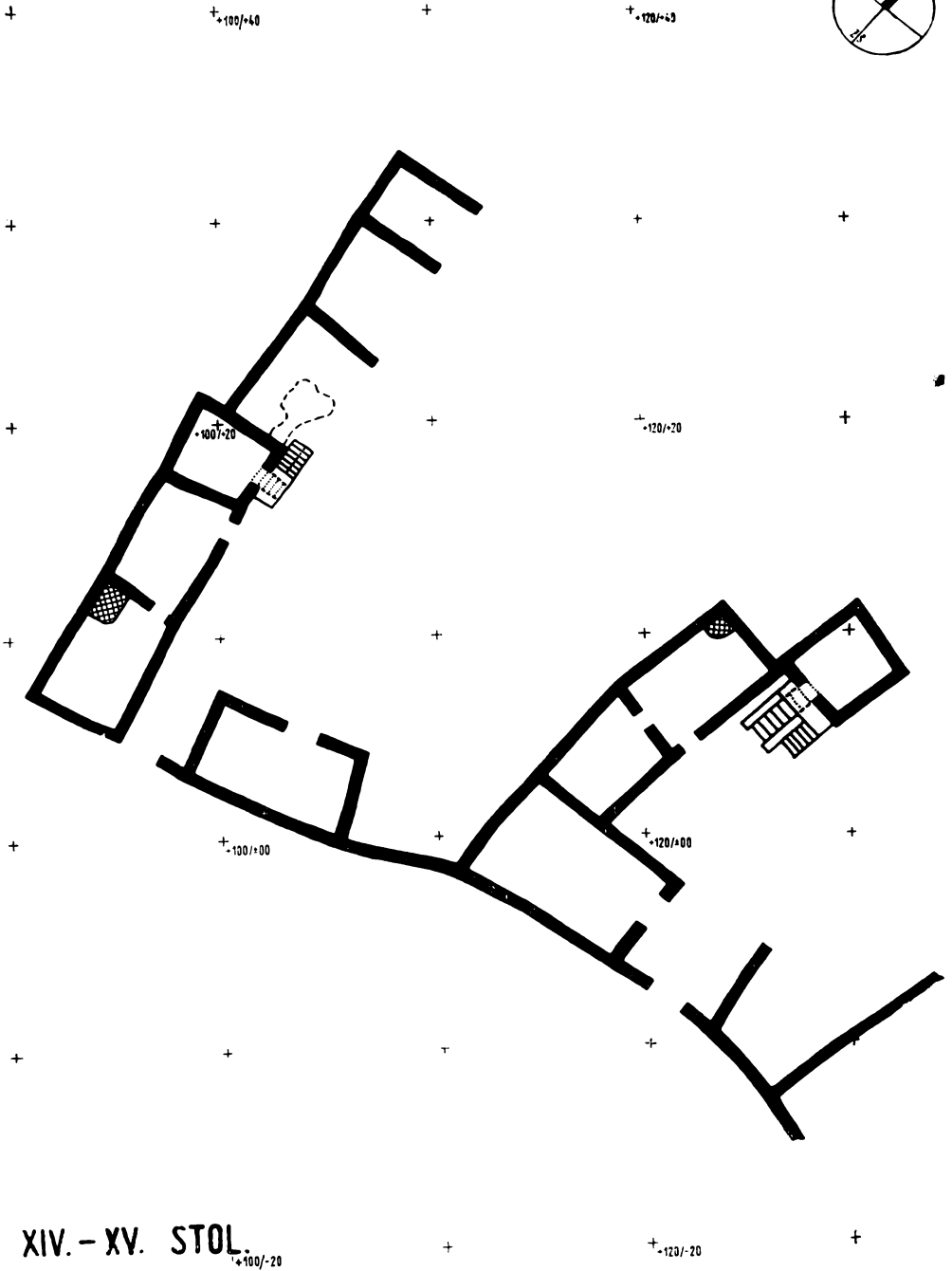
Obr. 3. Mstěnice. Půdorys usedlosti II/64 a III/71. Kresba ing. Z. Špičák.
