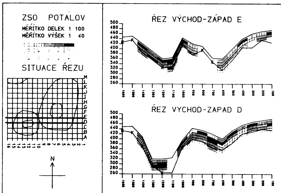
Obr. 9. ZSO Potálov, okres Tábor. Ukázka způsobu vykreslení vertikálního řezu terénem a předpokládané kulturní vrstvy s kameny a chlími se zakreslením koncentrací P_2O_5 . K – kámen, C – chlíva.
