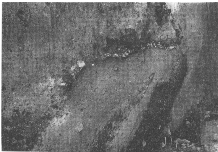
Obr. 2. Nahoře: Severní průkop valem, sonda II. Profil se střídajícími se vypálenými a nevypálenými vrstvami. Vzádu ve středu zřejmě jádro původního valu. – Dole: Severní průkop valem, sonda II. Detail s kamenitou vrstvou, zbytky spálených dřev a vypálený jíl.
