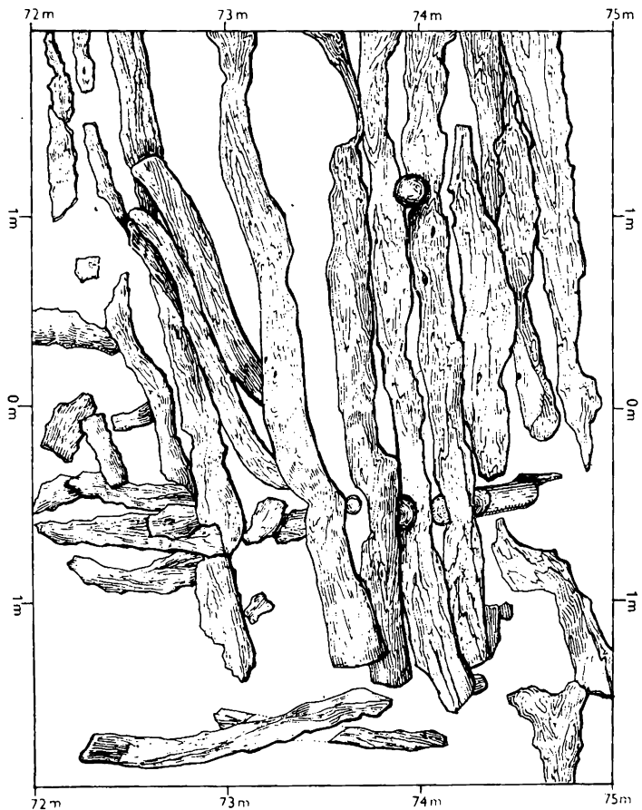
Obr. 4. Půdorys trámů na vnitřní straně valu. Sonda II. Měř. 1:20.
