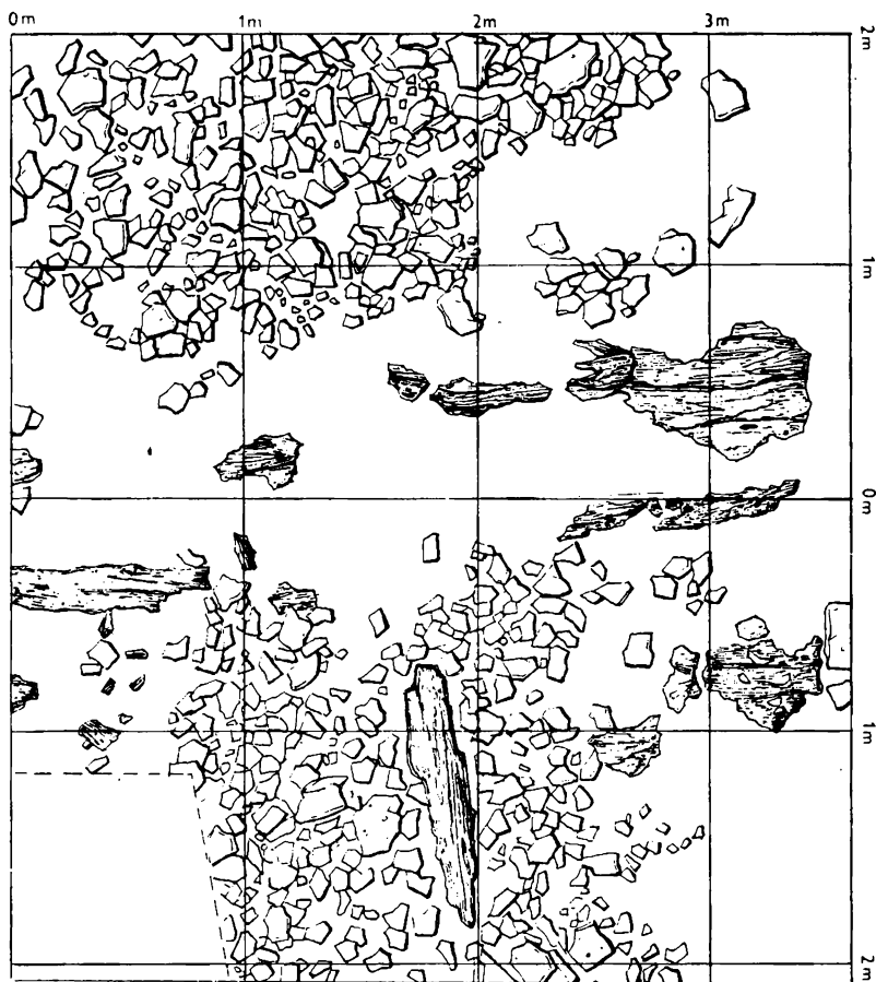
Obr. 5. Půdorys průřezu valem. Sonda II. Měř. 1:20.
