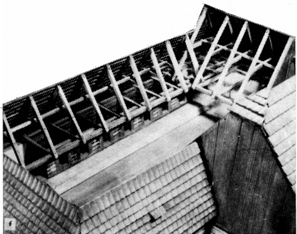
Obr. 2. d) Konstrukce krovů na nároží humenné podstáje a „starých chlévů“. e) Konstrukce krovů na nároží humenné podstáje a komory. f) Konstrukce krovů na nároží „starých chlévů“ a návěsní podstáje.
