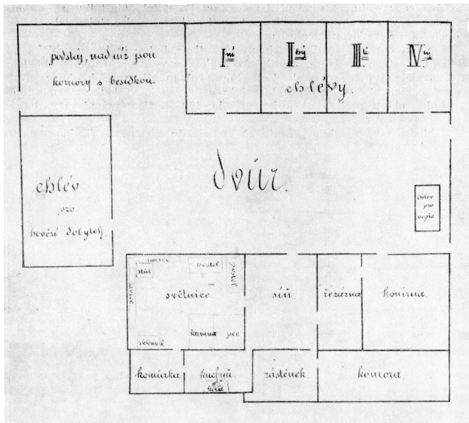
Obr. 6. Půdorys statku v Lazanech u Litomyšle č. 1.
