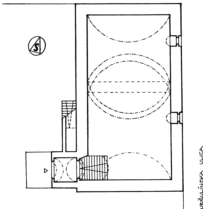
Obr. 18. Hypotetická rekonštrukcia domu z 2. pol. 13. st. Pôdorys dolného podlažia.
