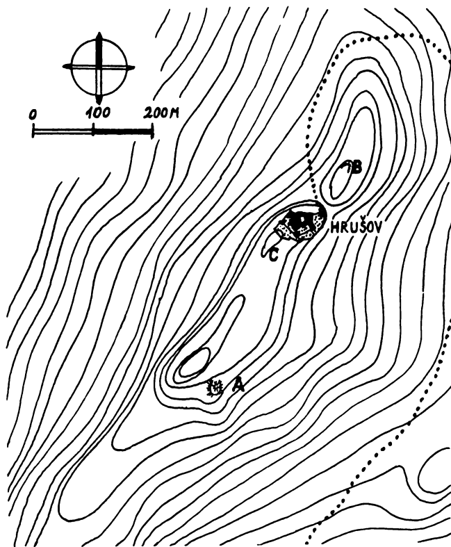
Obr. 1. Situácia hradu Hrušov s okolitými vyvýšenými polohami a prístupovou komunikáciou.
