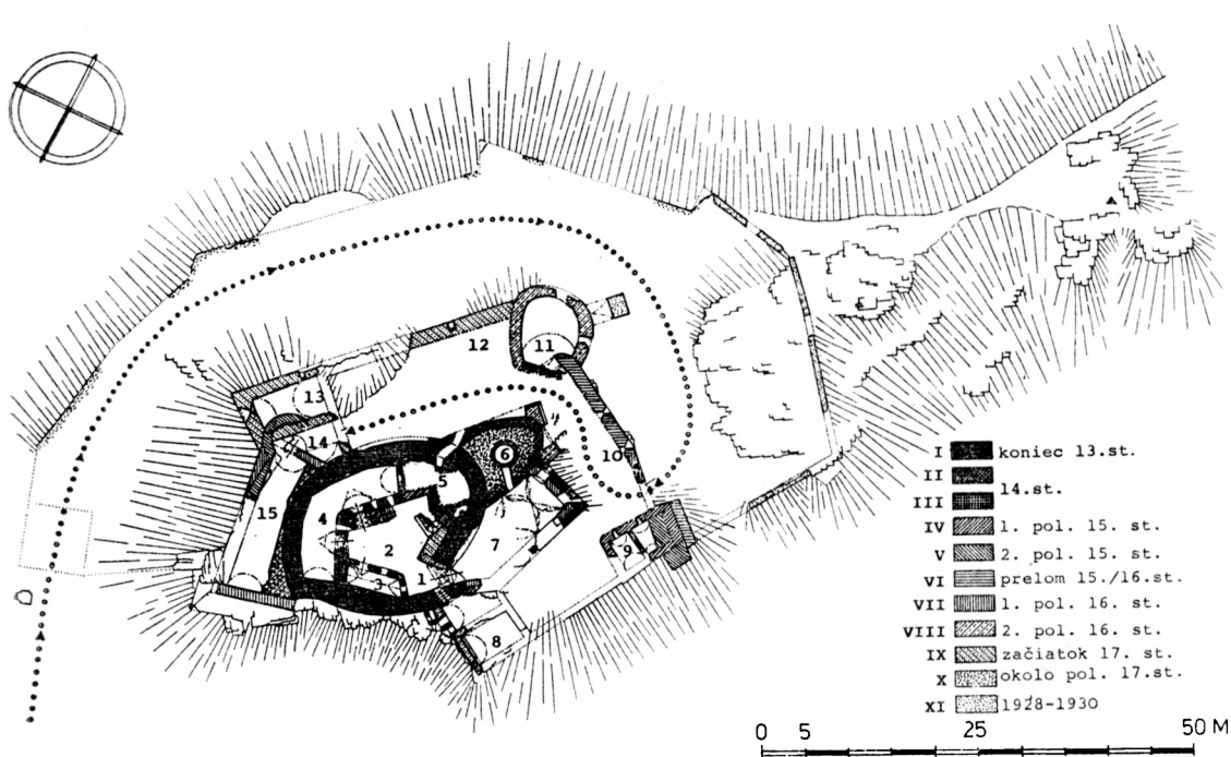
Obr. 3. Pôdorysné zameranie hradu Hrušov s vyznačením stavebných etáp (prízemia objektov).
