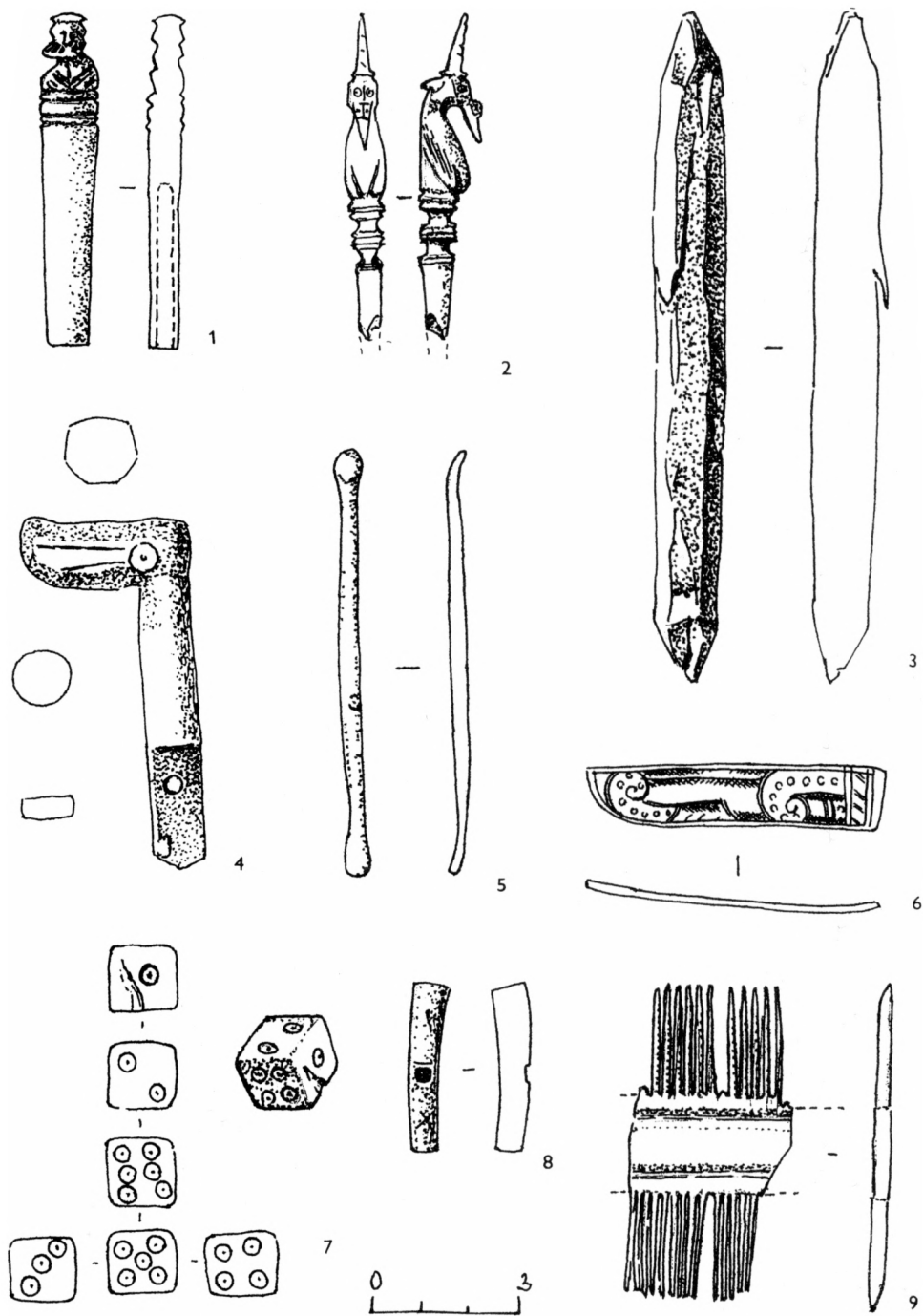
Obr. 8. Výrobky z kostí. Kresba J. Patsch.
