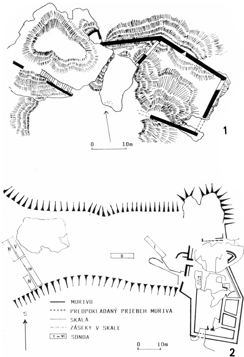
Obr. 2. Pôdorys stredovekého hradu, situácia v časoch A. Kmet'a (1) a v r. 1978 (2). Kresba autor.
