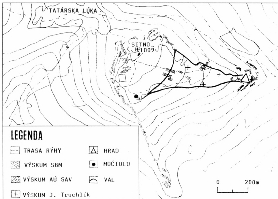
Obr. 1. Pôdorys lokality. Kresba autor.
