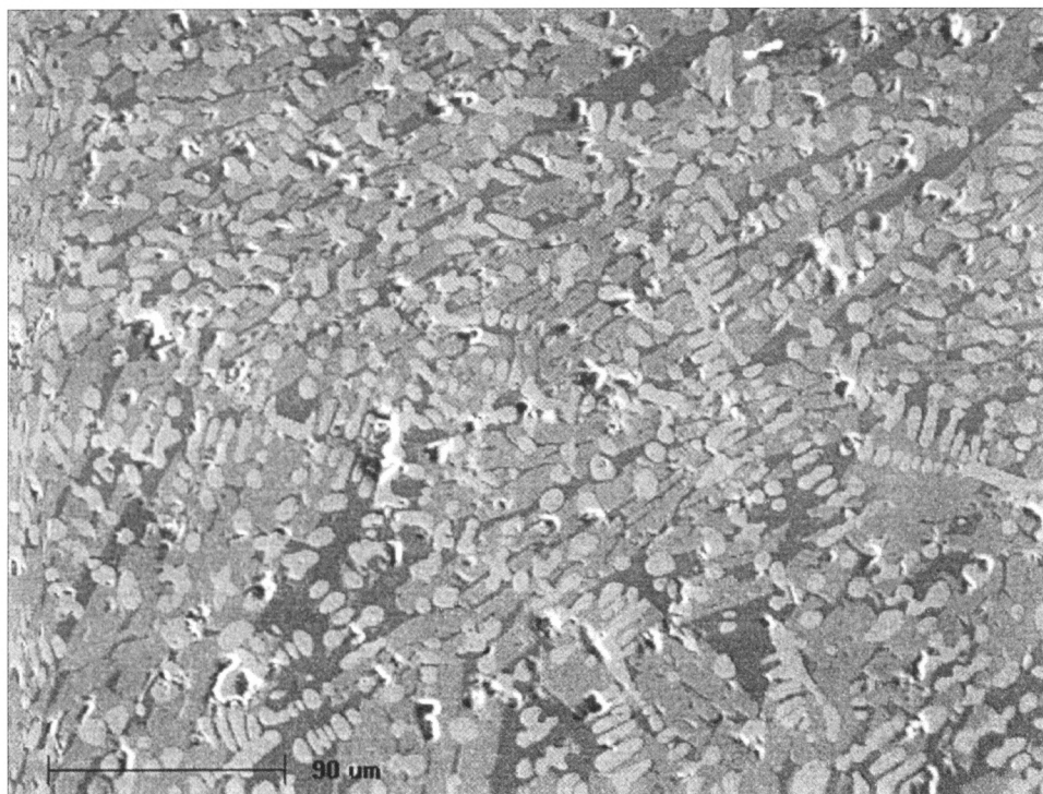
Obr. 8. Čáslav (okr. Kutná Hora), Střední průmyslová škola. Hutnická struska s wustitem (světlý), fayalitem (šedý) a K-sklouvinou (tmavošedá), BSE, foto. Z. Korbelová.
