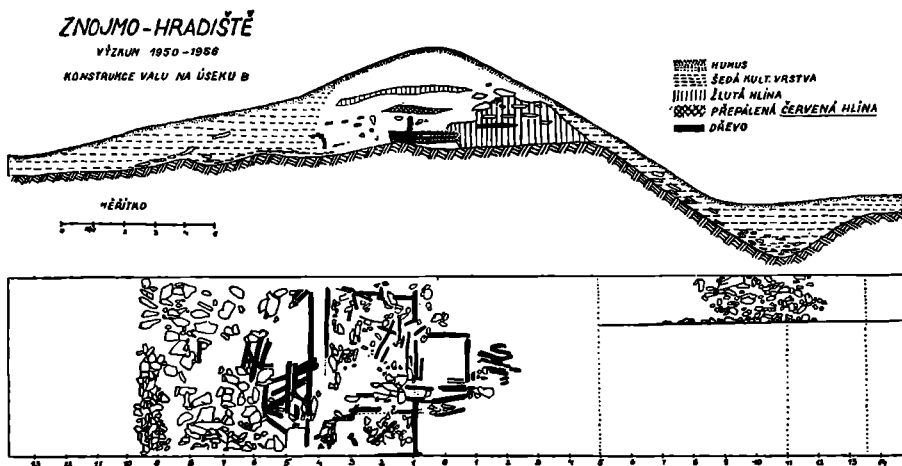
Obr. 10. Znojmo-Hradiště. Konstrukce opevnění. — Kresba: M. Havelka.
