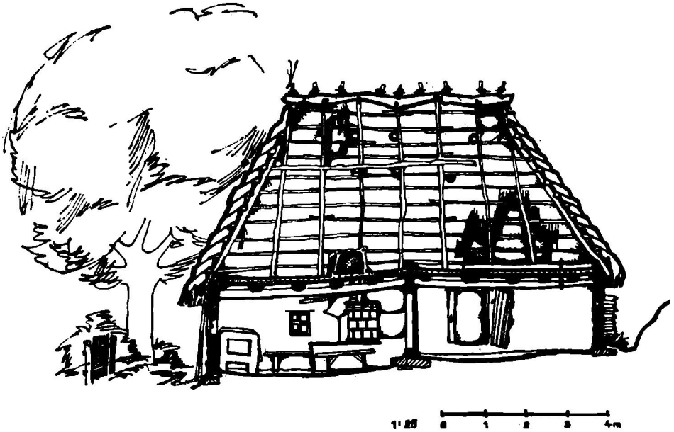
II. Zweiteiliges Haus, Lopeník, Nr. 118, Bez. Uherské Hradiště, 1946.
