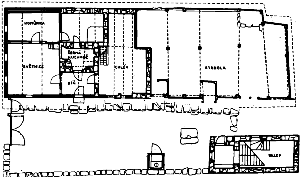
VIII. Mehrräumige Mischform des Bauernhauses, Čížov, Nr. 40, Bez. Znojmo, 1947.
