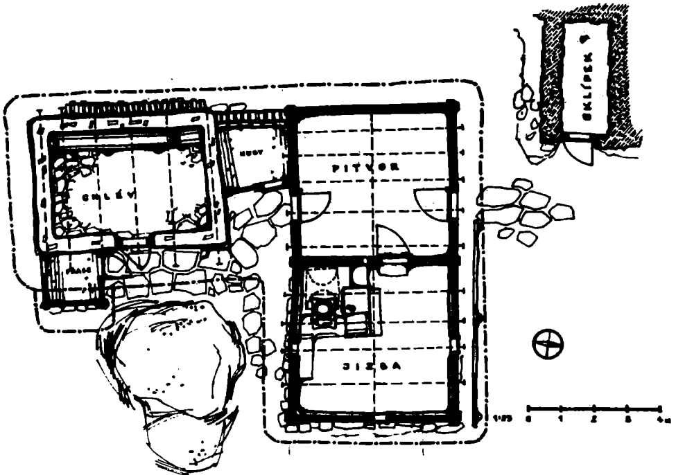
I. Zweiteiliges Haus, Lopensk, Nr. 118, Bez. Uherské Hradiště, 1946.
