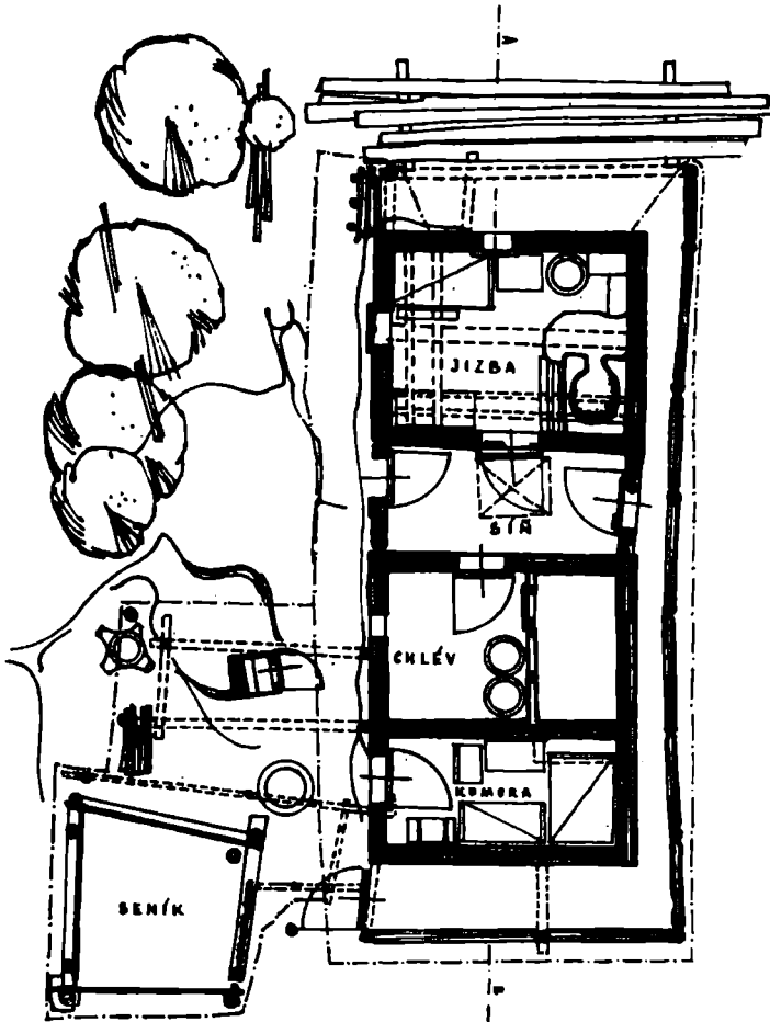
VI. Dreiteiliges Wohnstallhaus, Bukovec, Bez. Frýdek-Místek, 1946.
