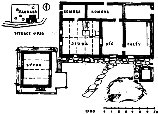
X. Mischform des Blockhauses, Horní Lideč, Nr. 18, Bez. Vsetín, 1963.
