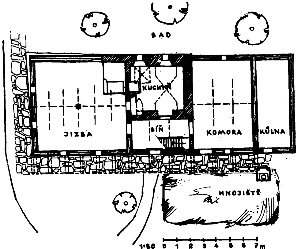
V. Dreiteiliges Wohnspeicherhaus mit der schwarzen Küche, Jasenná, Nr. 60, Bez. Gottwaldov, 1963.
