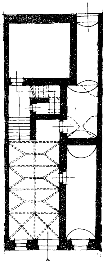
4. Moravská Třebová, náměstí č. 30, půdorys přízemí.
