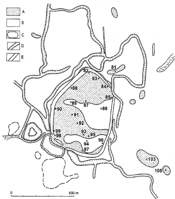
Obr. 49 – Pohansko. Geologická situace na mapě 1:10 000 (podle Poláček et al. 2005), A – říční písky, B – povodňové hlíny, C – písčito-šterkovité sedimenty, D – zaniklá ramena, E – opevnění.
