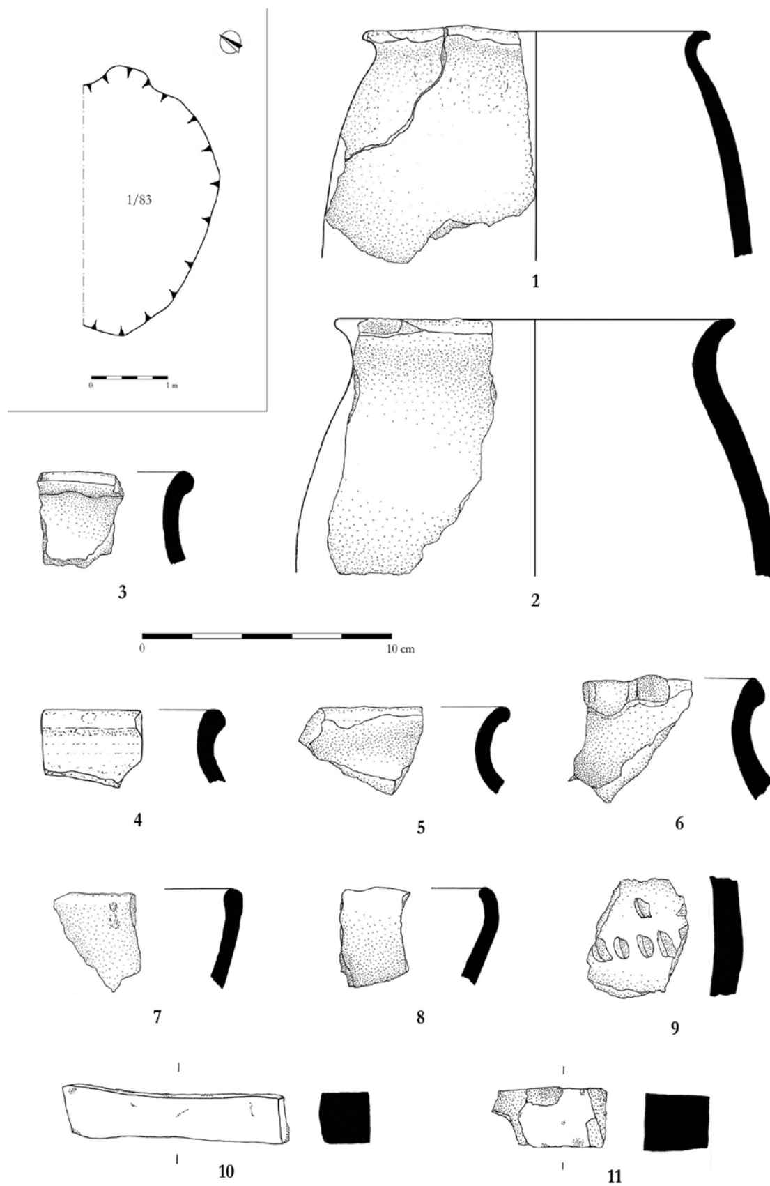
Obr. 5. Dědice u Vyškova. Objekt 1/83. 1–9 keramika, 10–11 kámen. Kresby: P. Gottvald.
