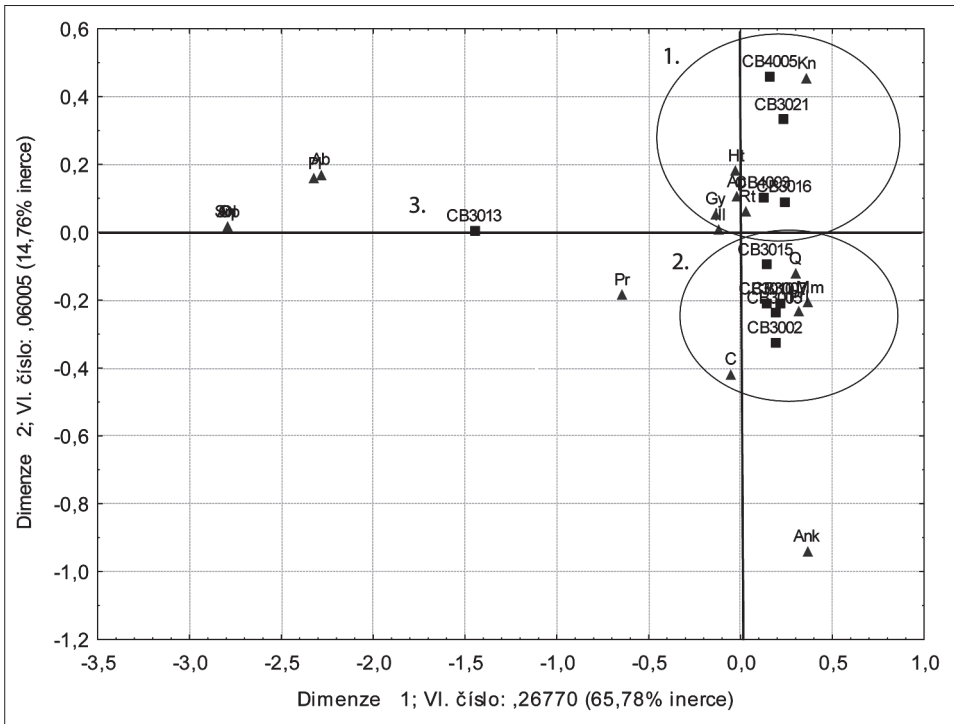
Obr. 7. Graf korespondenční analýzy. Vzájemné asociace mezi minerály a keramickými třídami. Rozlišené technologické skupiny 1 – převážně redukční keramika, 2 – grafitová keramika, 3 – třída CB3013 s neplastickými zrnky grafitu. Vytvořil L. Čapek. Abb. 7. Diagramm einer Korrespondenzanalyse. Assoziierung zwischen Mineralien und Keramikklassen. Technologisch differenzierte Gruppen 1 – überwiegend Reduktionskeramik, 2 – Graphitkeramik, 3 – Klasse CB3013 mit nichtplastischen Graphitkörnern. Erstellt von L. Čapek.
