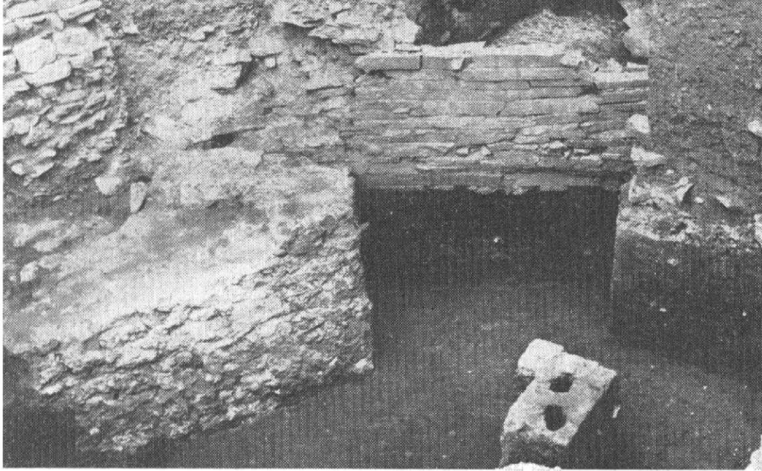
Obr. 1. Olomouc – dómské návrší 1983: Jihovýchodní nároží podélné orientované stavby (kaple sv. Máří Magdaleny?) a kamenná plenta na vnitřní straně mladohradištního valu. Za plentou jílová báze valového násypu. Foto: V. Bittner.
