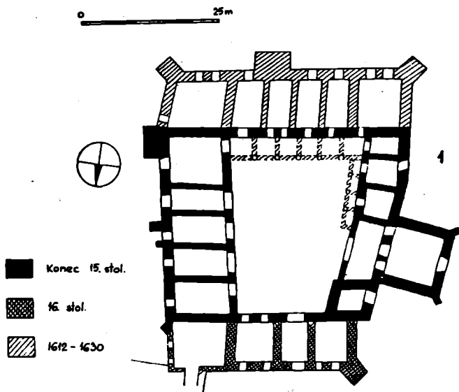
Obr. 4. Moravská Třebová (okr. Svitavy). Vývojové schéma jádra zámku (podle Z. Kudělnky).
