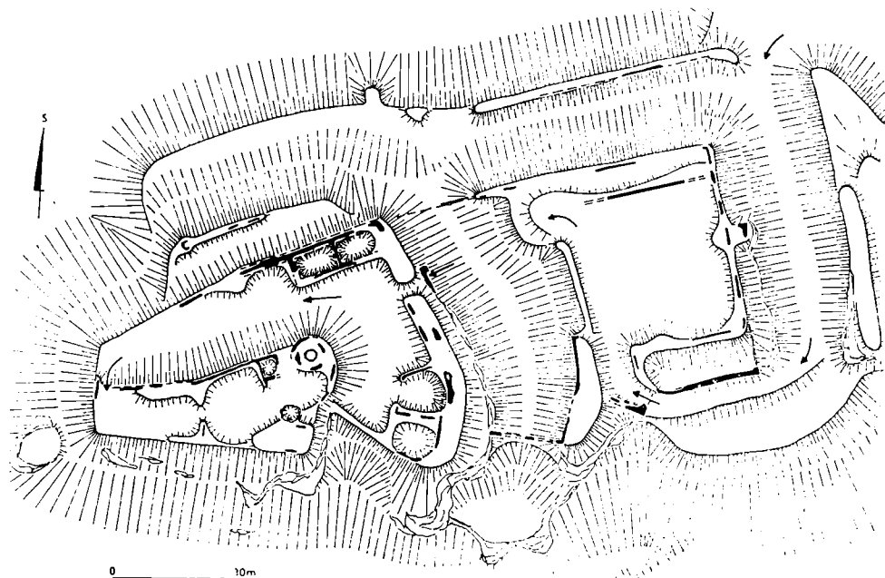
Obr. 6. Dolní Loučky (okr. Žďár n. Sáz.). Příklad pozdně gotického předhradí se vstupním koridorem a štítovou zdí druhého předhradí.
