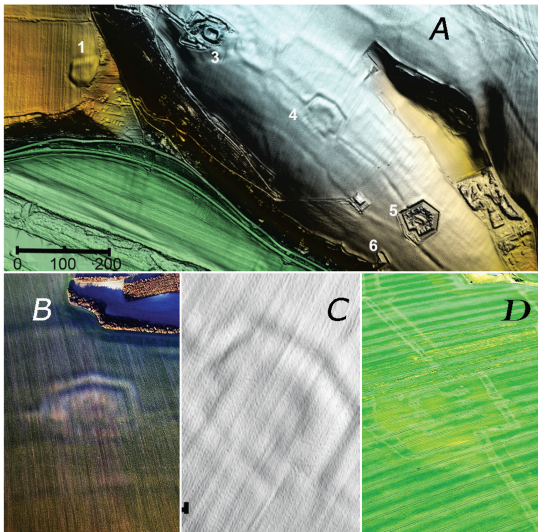
Obr. 2a. Dokumentace lokality – opevnění z poloviny 19. stol. poblíž Litoměřice – dokumentované tradičním způsobem, resp. šikmými fotografiemi (B – stínové příznaky, D – vegetační příznaky) a leteckým laserovým skenováním (A, C – stínovaný digitální model terénu).
