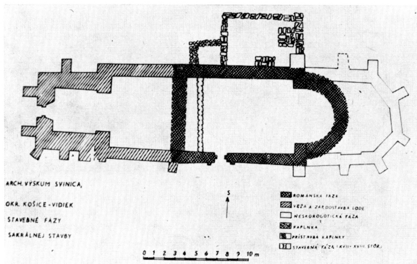
Obr. 6. Svinica, okr. Košice-vidiek. Stavebné fázy sakrálnej stavby.
