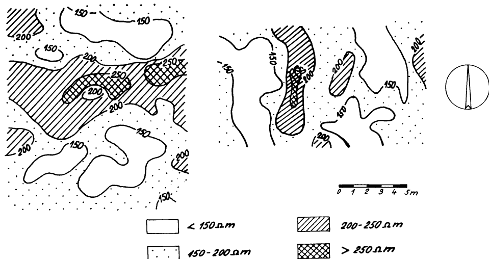
Obr. 13. ZSO Žárek u Sudoměřic (okres Tábor) — tvrz — geofyzikální zaměření. Zaměřil: Dr. V. Bárta.
