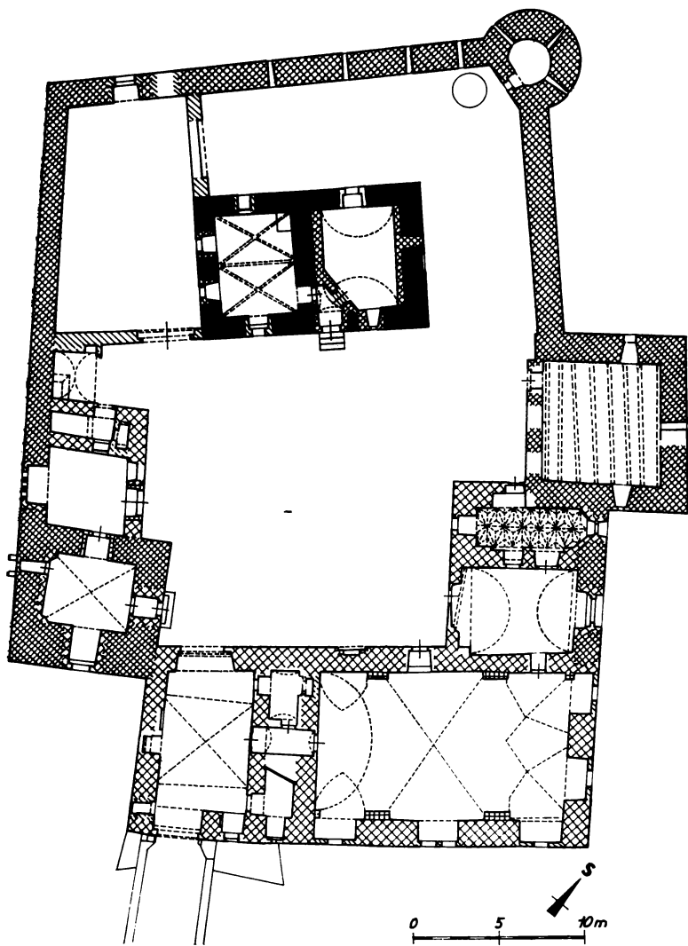
Obr. 2. Kestřany – půdorys přízemí Horní tvrze ve stavebně historické analýze, stav r. 1986 – vybourání dodatečných příček a mezistropů. Černé značeno raně gotické zdivo „purkrabství“ husté a řídké mřížky značí 2 pozdější gotické fáze, ostatní zdivo je renesanční a mladší. (F. Kašíčka)
