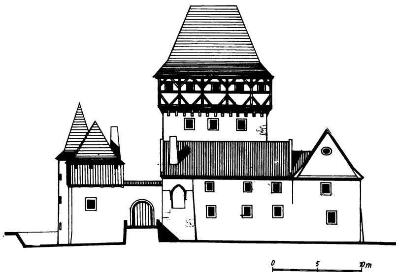
Obr. 5. Kestřany – čelní průčelí Dolní tvrze před započatím zabezpečovacích prací a rekonstrukce po-doby v 16. stol. (F. Kašíčka)
