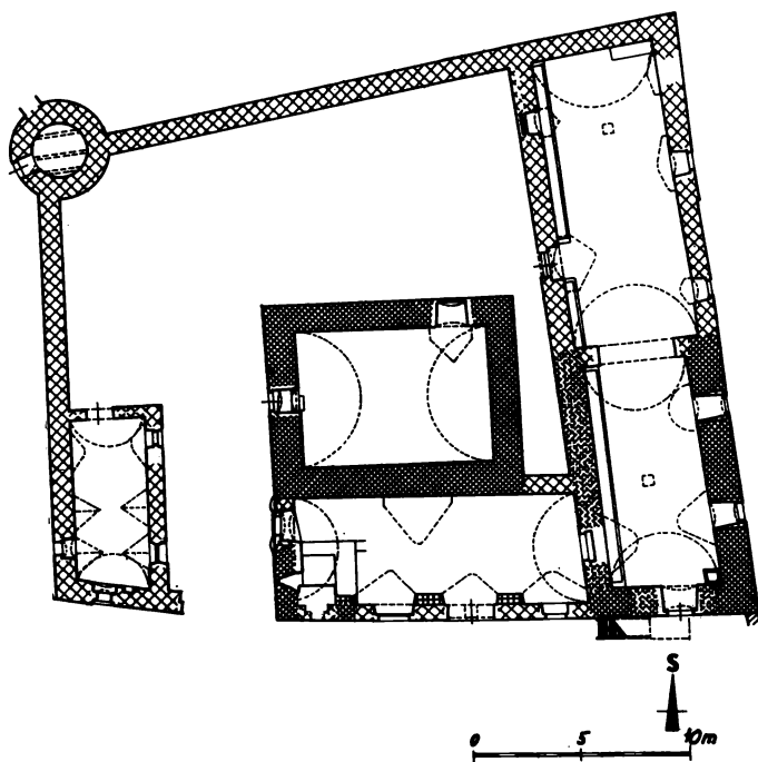
Obr. 4. Kestřany – půdorys přízemí Dolní tvrže ve stavbě historické analýze, stav 1986. Husté a řídké mřížky značí 2 gotické stavební fáze, ostatní zdívo je renesanční a mladší. (F. Kašíčka)
