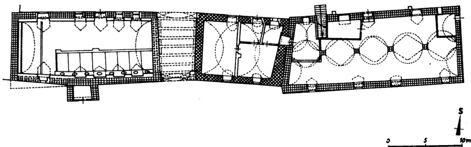
Obr. 6. Kestřany – přední hospodářské budovy, půdorys přizemí ve stavebně historické analýze. Šikmé mřížky značí zdívo gotické, mřížky kolmé ke konstrukci – renesanční, ostatní míčdiší. Přerušovaná šra-fura označuje zařazení hypotetické. (F. Kašíčka)
