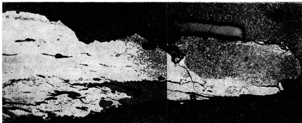
Obr. 15. Příčný řez bítím srpů.
