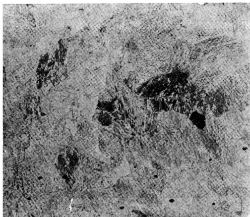
Obr. 16. a — příčný řez bítu sekery; b — jádro sekery; c — ukončení oduhličené vrstvy sekery; d — detail bítu sekery; e — rozhraní nauhličené vrstvy a jádra.
