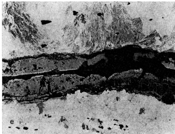
Obr. 16. a — příčný řez bítu sekery; b — jádro sekery; c — ukončení oduhličené vrstvy sekery; d — detail bítu sekery; e — rozhraní nauhličené vrstvy a jádra.
