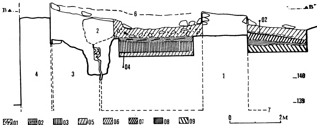
Obr. 4. Bratislava, Vodná veža. Stavba terénu pod základovou škárou muriva 6. fázy. Číslovanie pre- vzaté z výskumovej dokumentácie. 1-4, 6 - číslovanie zhodné s obr. 2, 7 - niveleta terénu v dobe výstavby oktogonu. 01 - deštruktívna vrstva z kamenného muriva, 02 - prepálený horizont, v interiéri veže s trámami a krytinou, 03, 05, 06, 09 - piesčitohlinité navážky, 04 - maltová kryha, 07, 08 - vrstva drobnej sute a malty z kamenného muriva.
