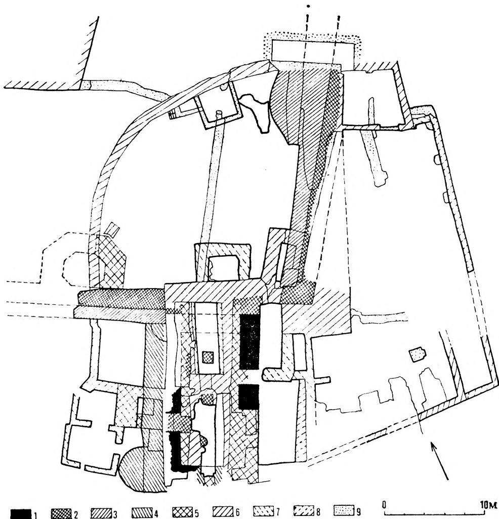
Obr. 1. Bratislava, Vodná veža. Celková situácia oktogonu v prevzatej stavebnohistorickej analýze. V. Ferusa a K. Klínčokovej s predbežnou synchronizáciou s 5. stavebnou etapou. 1 – doba rímska, 2 – 11. až zač. 12. stor., 3 – 12. stor., 4 – koniec 12. až zač. 13. stor., 5 – okolo pol. 13. stor., 6 – po r. 1361, 7 – prvá pol. 15. stor., 8 – prvá pol. 16. stor., 9 – po pol. 17. stor.
