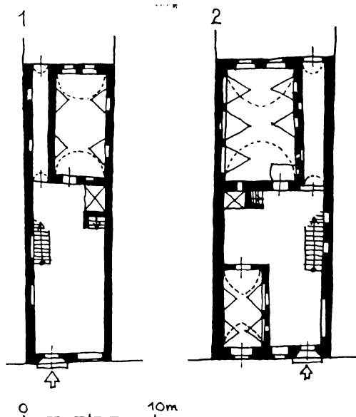
Obr. 10. Warszawa — Síňové domy ze 16. století, ulice Nowomiejská č. 9 a č. 5 s vestavěným kontorem.
