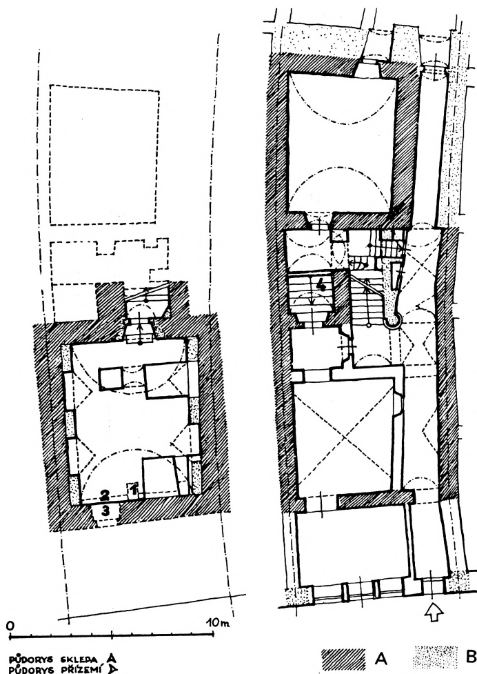
Obr. 11. Mladá Boleslav — dům čp. 16, původně síňový. A — V nejstarší zděné fázi výstavby domu se uplatňují pozdně-gotické architektonické detaily. Nemí však vyloučeno, že zadní polozapuštěná komora a snad i obvodové zdi jsou staršího původu. Síň, polozapuštěná komora a přední sklep byly plochostropé. V předním sklepe se zachovala část průvlaku (1) a trám původního plochého stropu (2). V čelní stěně je patrný vstup ke sklepní špi (3). B — Při renesanční přestavbě byl zaklenut přední sklep a zbudováno zděné schodiště do mezipatra a patra. Patro bylo předsunuto na představené zděné loubí. Síň zůstala až do barokní přestavby plochostropá. Charakteristický přístup do sklepa ze síně (4) zůstal ve funkci až do 19. století.
