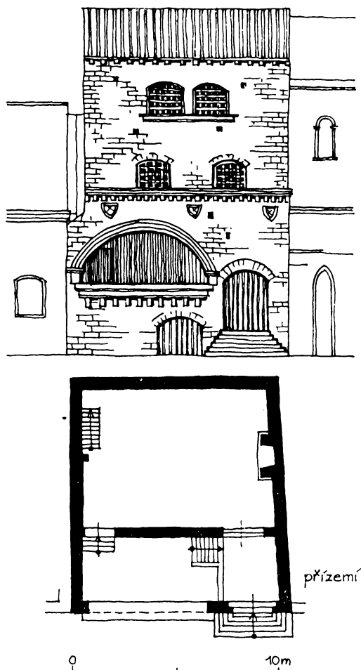
Obr. 5 Viterbo — dům církevního hodnostáře na Piazza San Pellegrino, 13. stol.
